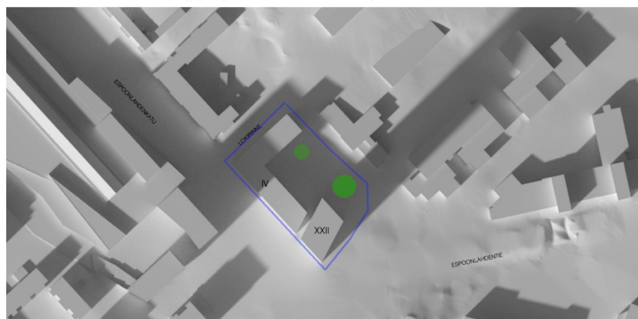
tilanne 20.9. (syyspäivän tasaus) klo 15
