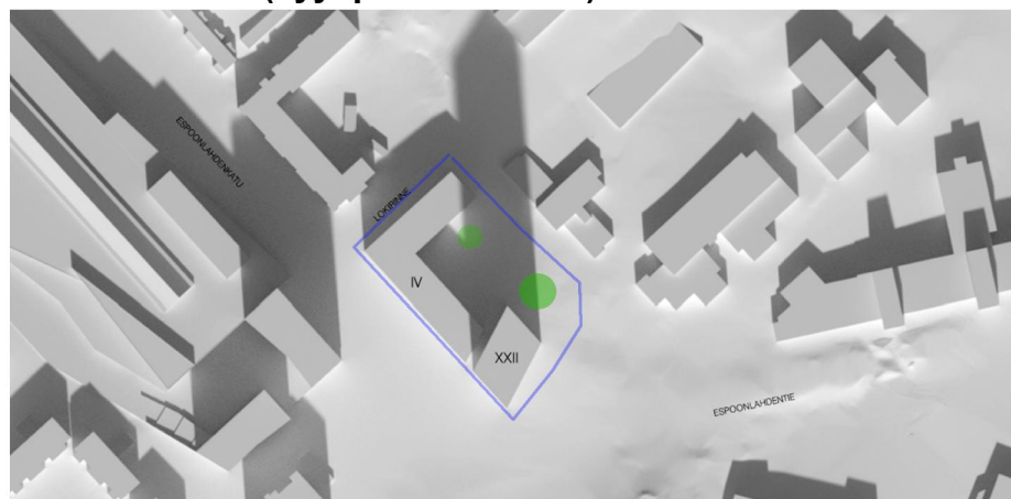
tilanne 20.9. (syyspäivän tasaus) klo 12
