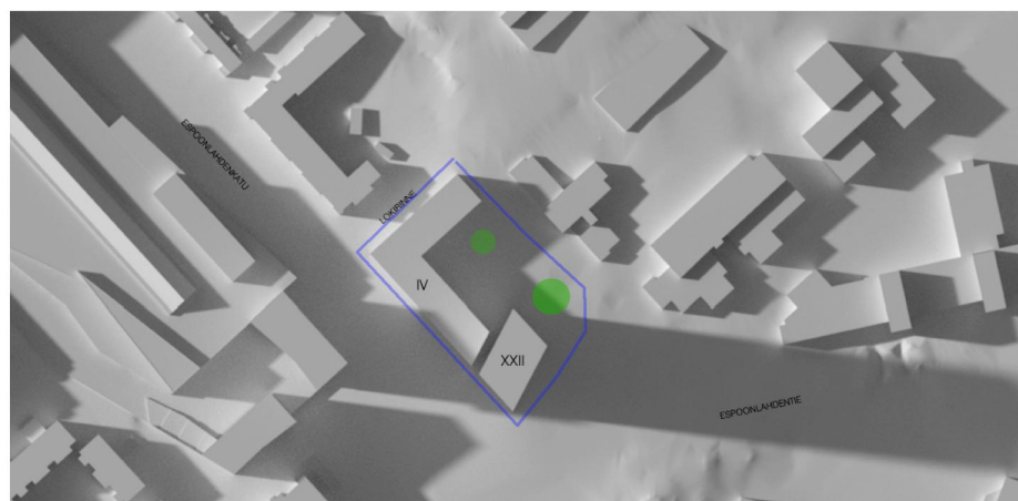
tilanne 20.9. (syyspäivän tasaus) klo 18
