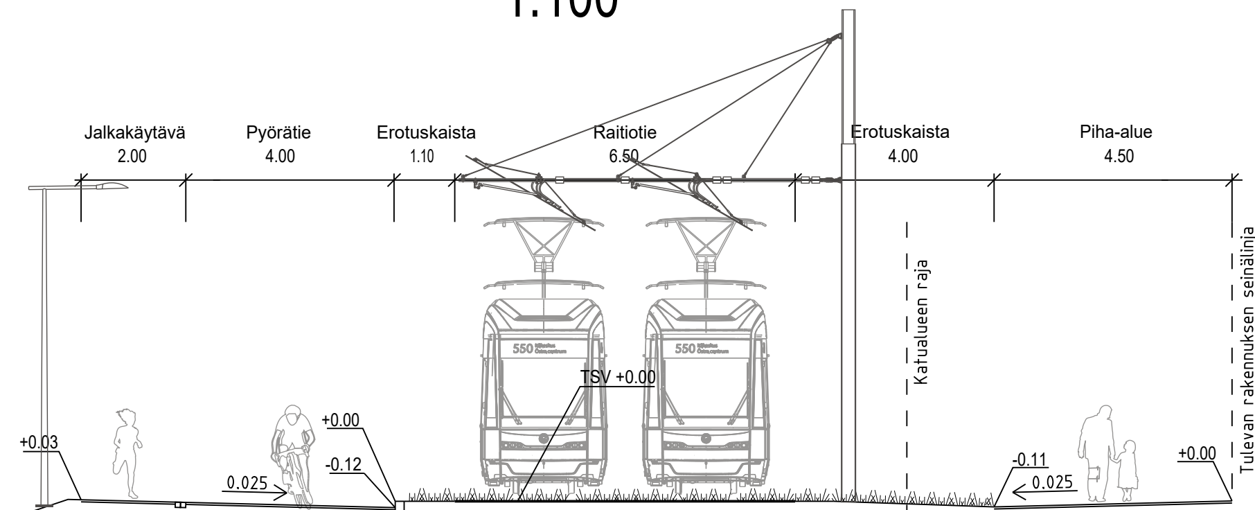
TYYPPIPOIKKILEIKKAUS B-B 1:100
