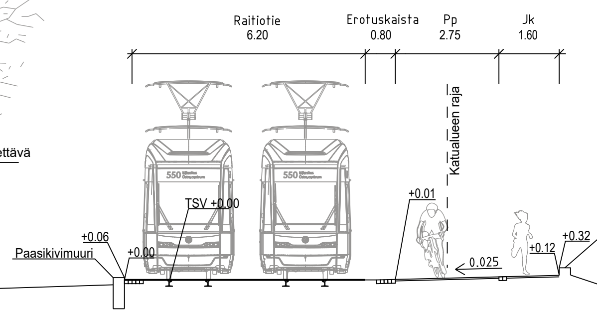
TYYPPIPOIKKILEIKKAUS B-B 1:100
