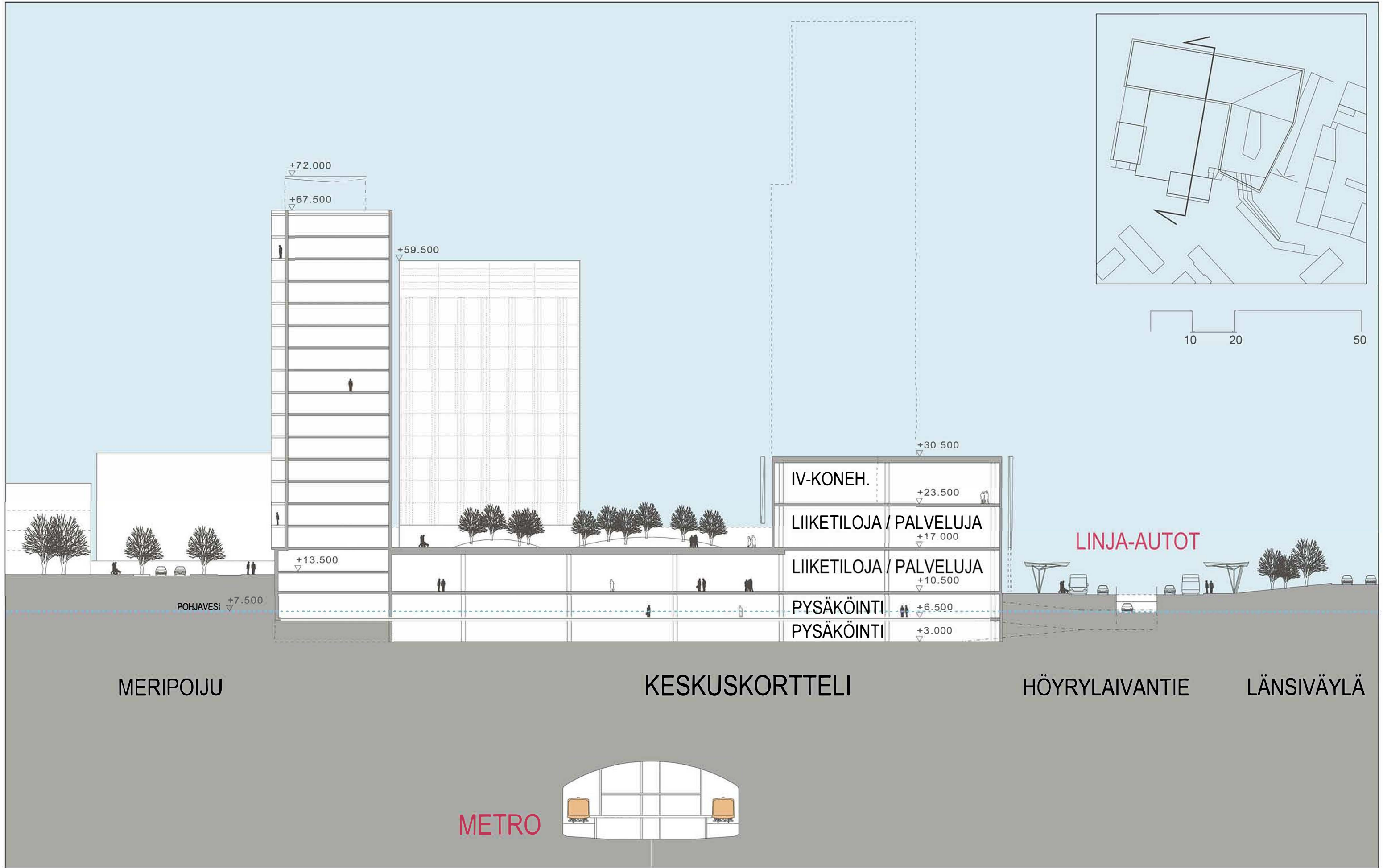
KIVENLAHDEN METROKESKUS LEIKKAUS C-C 1:500 KESKUSKORTTELI
