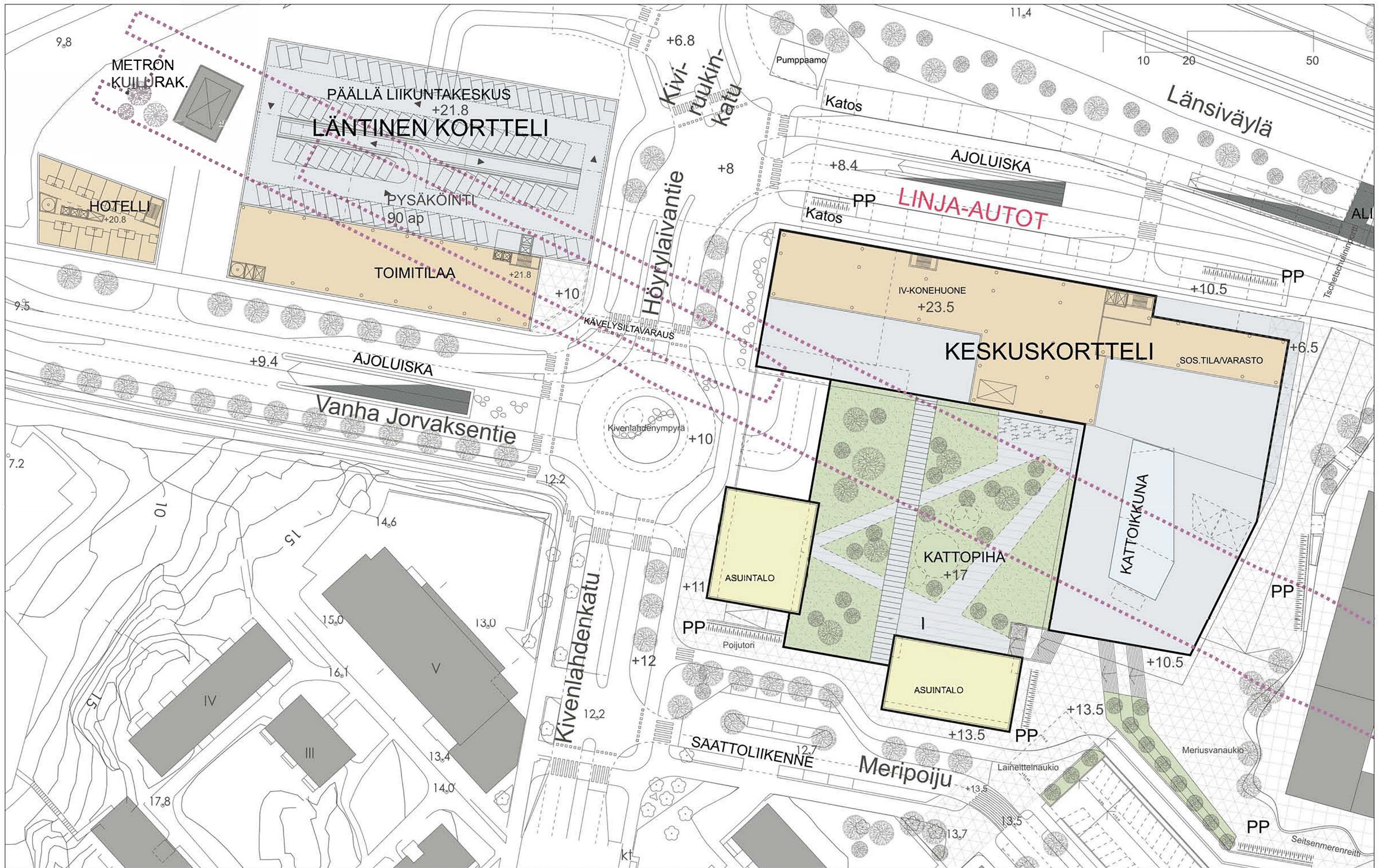
KIVENLAHDEN METROKESKUS POHJAPIIRUSTUS +23 1:800 KESKUSKORTTELI & LÄNTINEN KORTTELI
