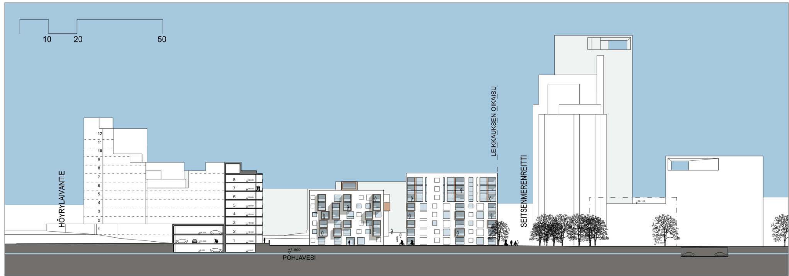
KORTTELILEIKKAUS A-A
