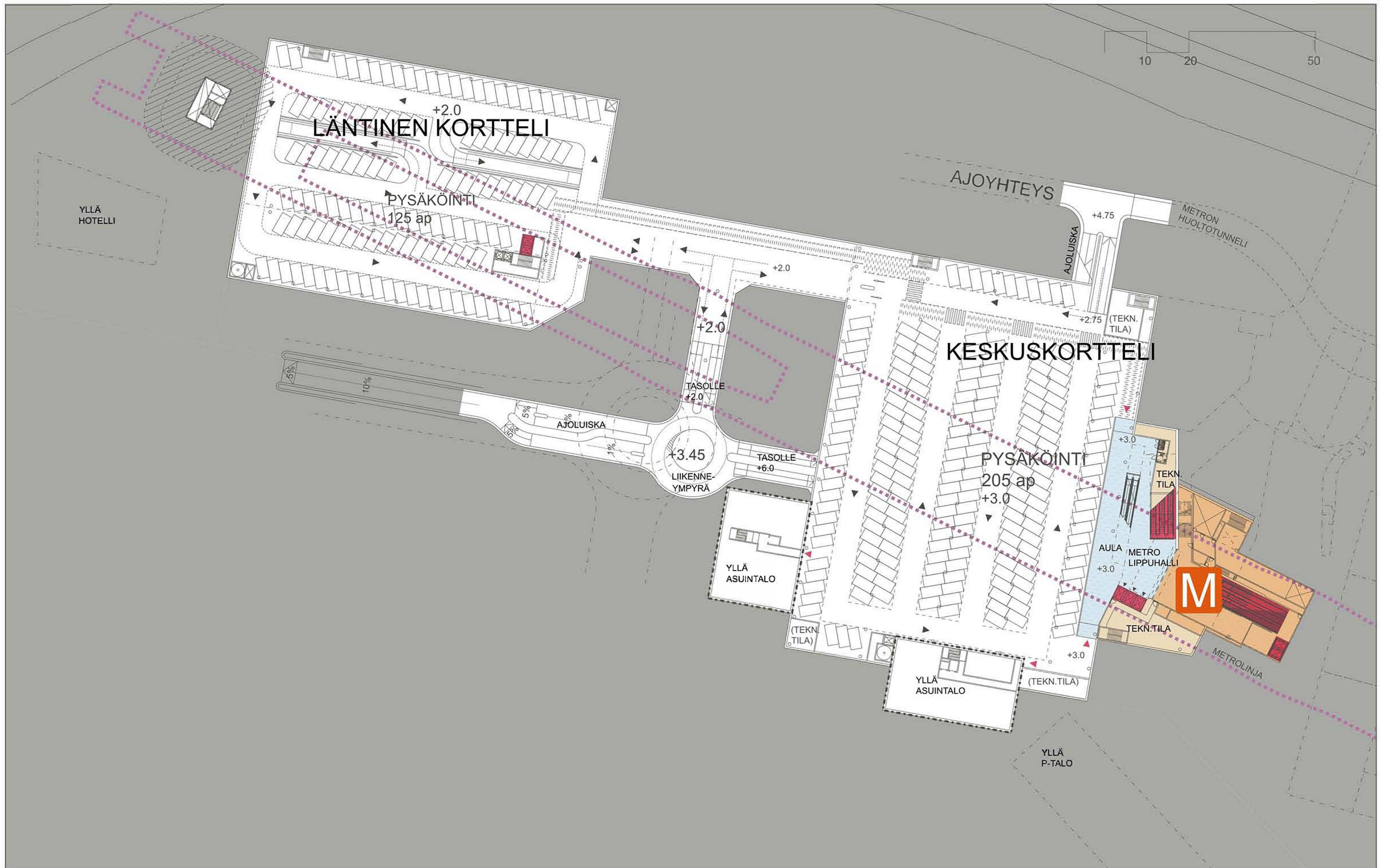
KIVENLAHDEN METROKESKUS POHJAPIIRUSTUS +3.0 1:800 KESKUSKORTTELI & LÄNTINEN KORTTELI
