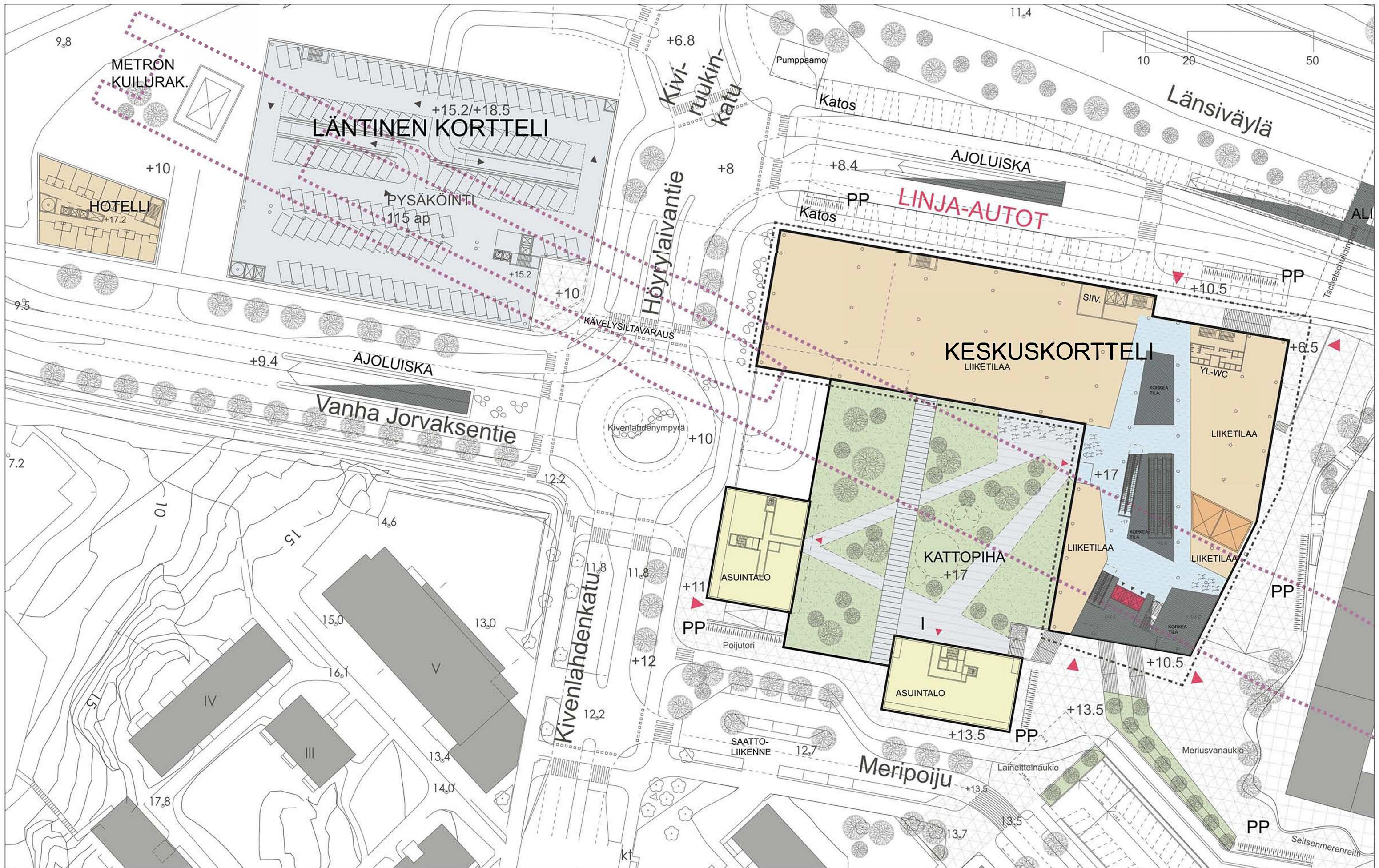
KIVENLAHDEN METROKESKUS POHJAPIIRUSTUS +17 1:800 KESKUSKORTTELI & LÄNTINEN KORTTELI
