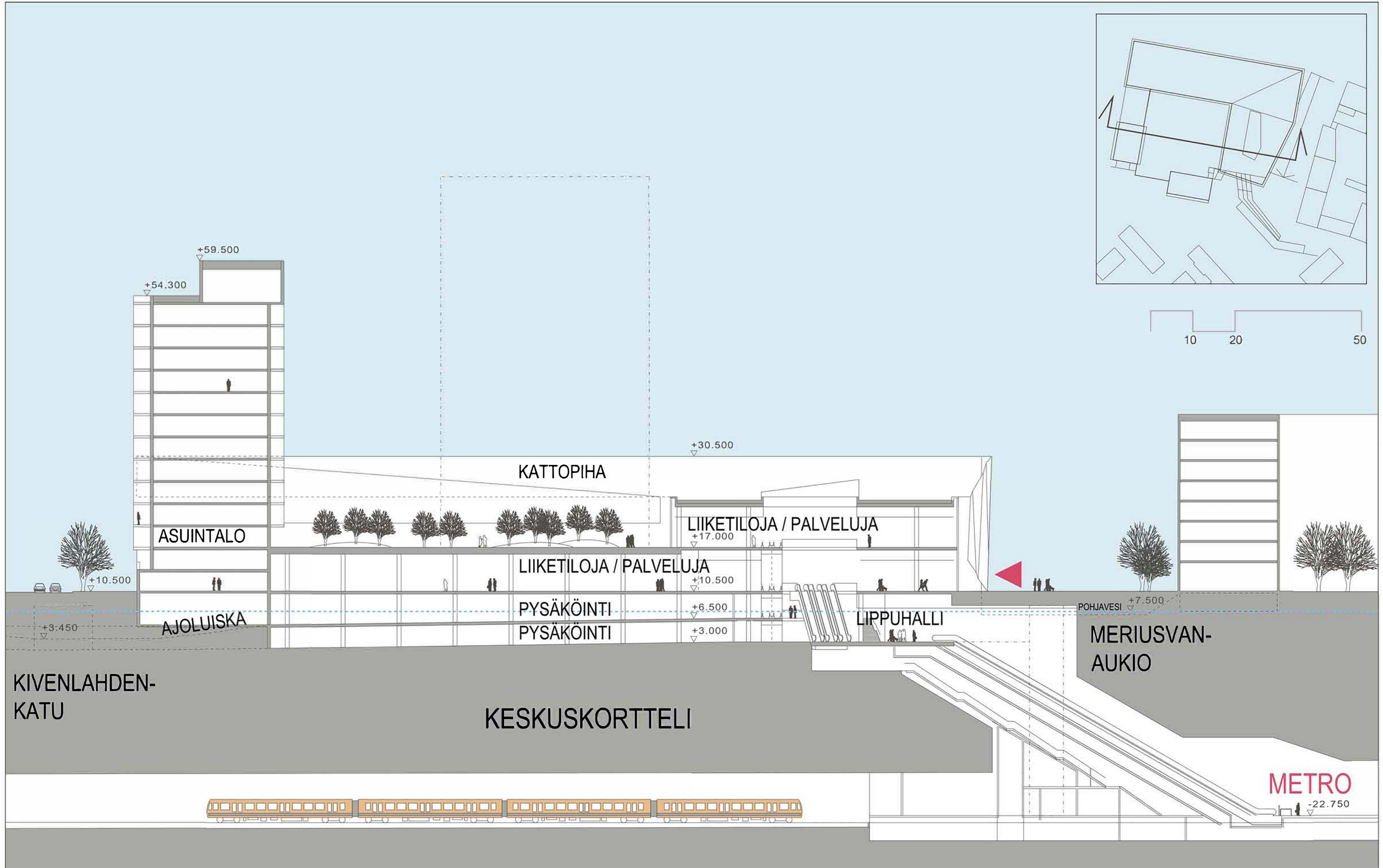
KIVENLAHDEN METROKESKUS LEIKKAUS B-B 1:500 KESKUSKORTTELI
