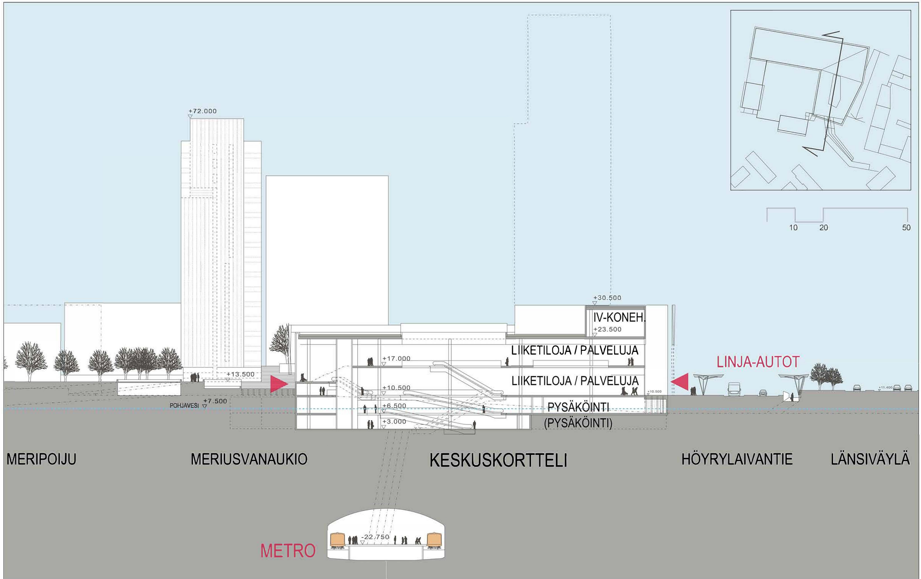
KIVENLAHDEN METROKESKUS LEIKKAUS A-A 1:500 KESKUSKORTTELI
