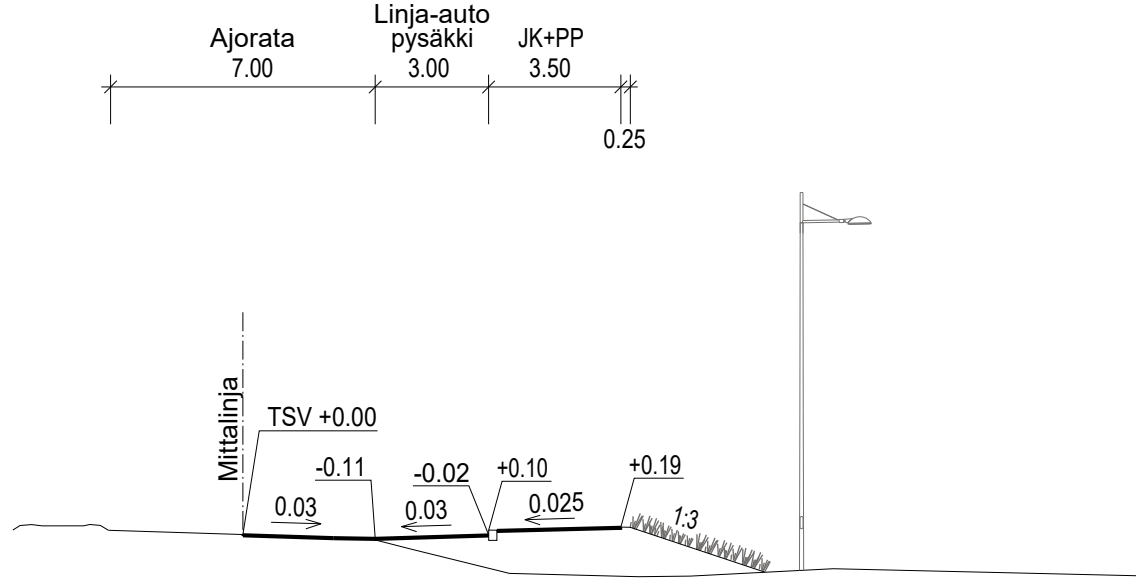
TYYPPIPOIKKILEIKKAUS C-C 1:200
