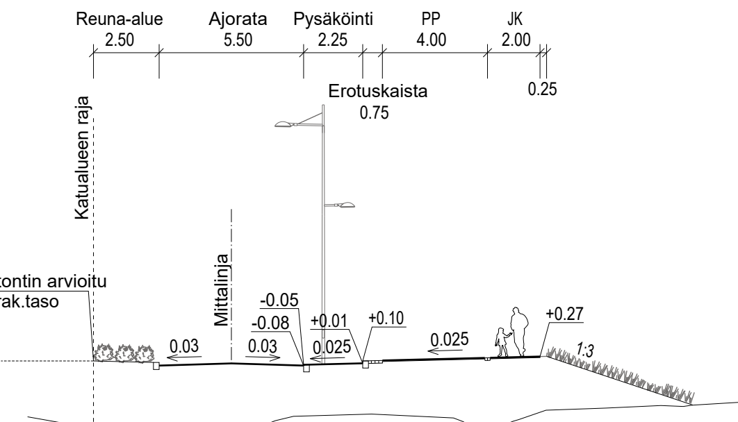
TYYPPIPOIKKILEIKKAUS A-A 1:200
