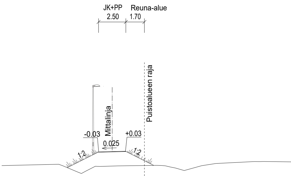
TYYPPIPOIKKILEIKKAUS B-B 1:200
