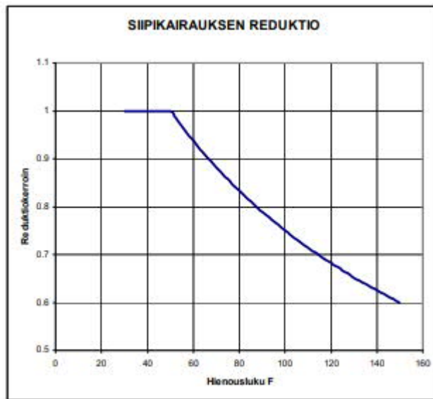
Kuva 2. Siipikairauksen leikkauslujuuden reduointi hienousluvun mukaan (Liikennevirasto, Penkereiden stabiileetin laskentaohje 14/2018, sivu 12)
