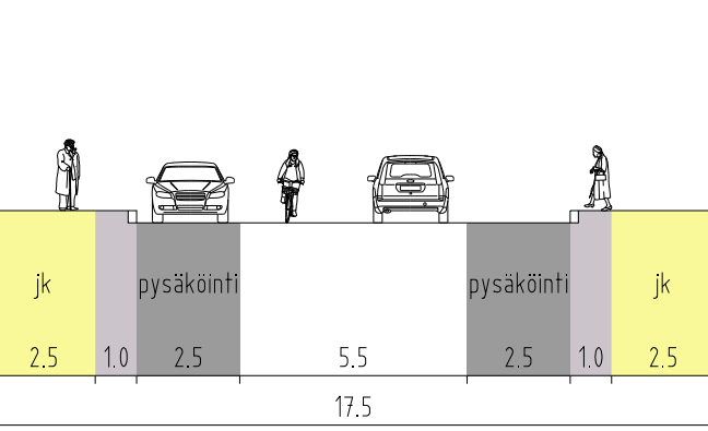
TERMINAALI + ASEMANRANTA, LEIKKAUS J - J
