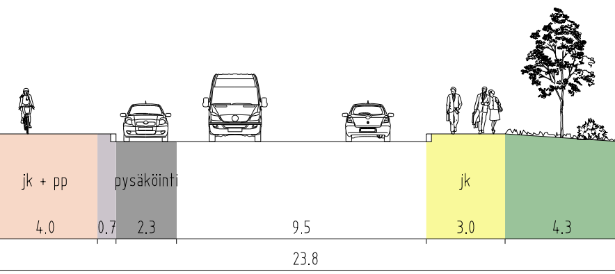
KATKAISIJANKATU, LEIKKAUS L - L
