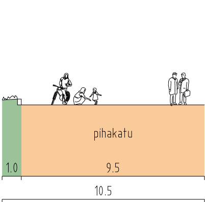
PUHALTAJANPOLKU, LEIKKAUS N - N
