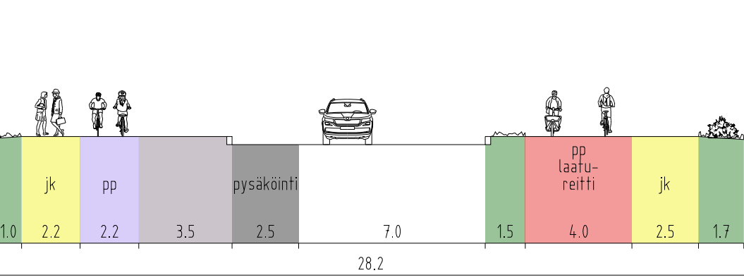
LILLBASSINKATU, LEIKKAUS E - E
