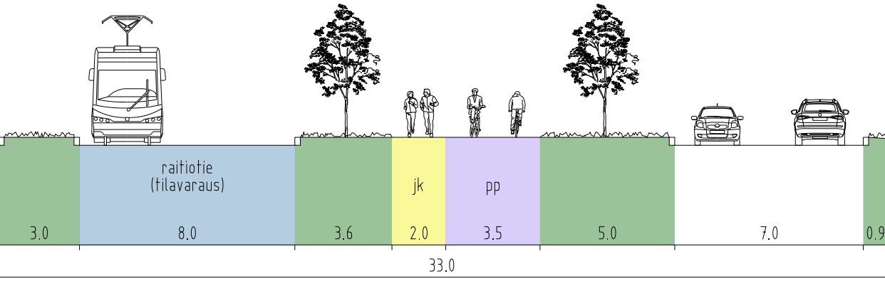
PUHALTAJANPOLKU, LEIKKAUS N - N
