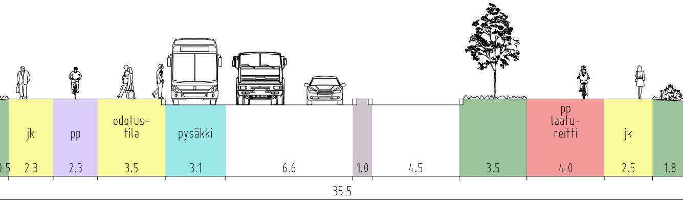
KANTAJANKATU, LEIKKAUS D - D
