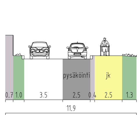
TAMARA BRUUNIN KATU, LEIKKAUS P - P
