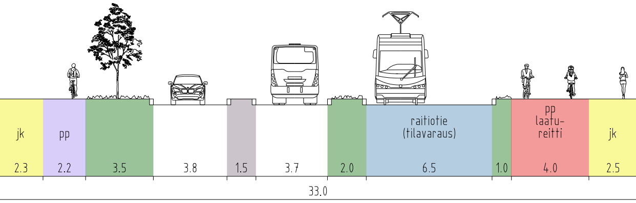
VANTINMÄENTIE, LEIKKAUS I - I
