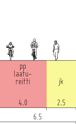
LILLBASSINREITTI, LEIKKAUS G - G
