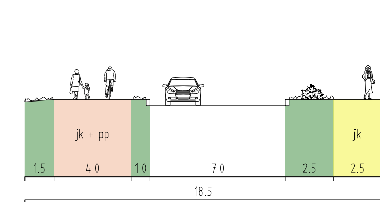
TAMARA BRUUNIN KATU, LEIKKAUS P - P
