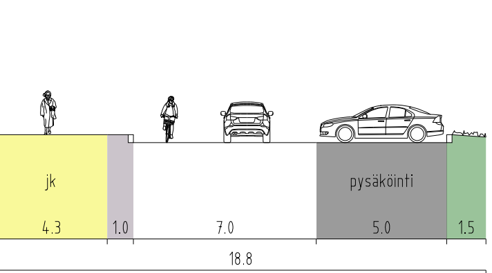
ALOITTAJANKATU, LEIKKAUS H - H
