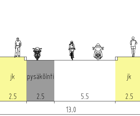
HYTTIMESTARINPOLKU, LEIKKAUS O - O
