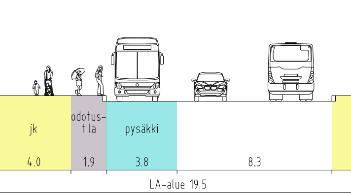
PUHALTAJANKATU, LEIKKAUS K - K
