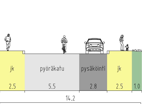
LILLBASSINKATU, LEIKKAUS F - F
