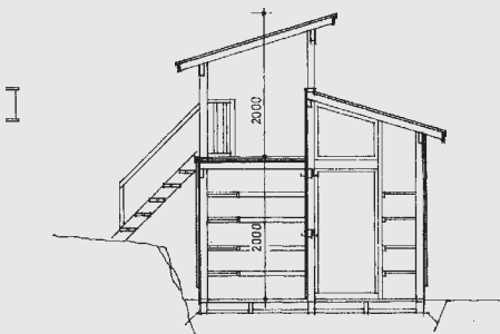
LEIKKAUS A-A
