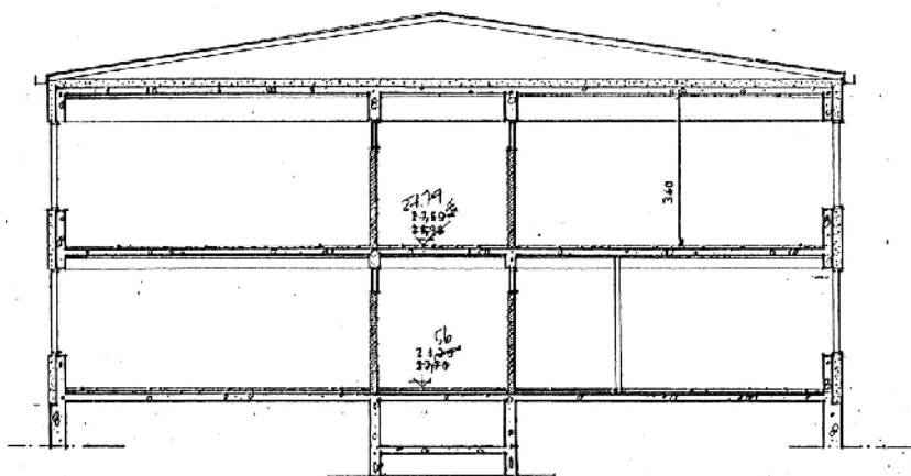
Leikkauspiirustus yläkoulusiiven kohdalta.
