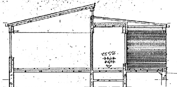
LEIKKAUS B-B
