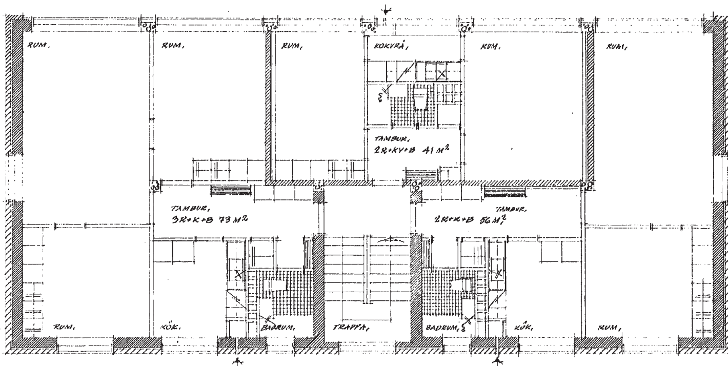
1. ja 2. kerroksen pohjapiirros
