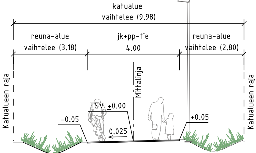
TYYPPIPOIKKILEIKKAUS A-A 1:100
