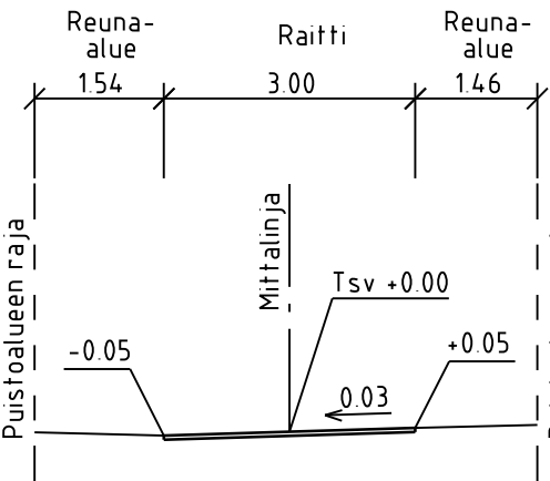
TYYPPIPOIKKILEIKKAUS A-A
