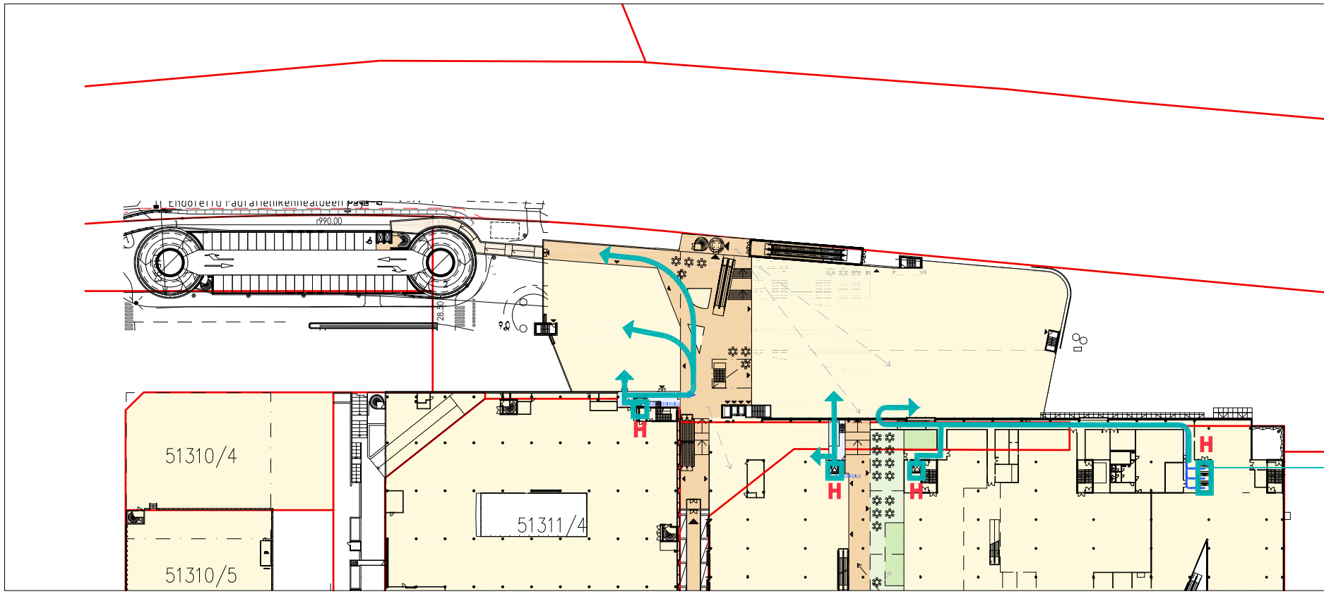
YHTEYDET SELLON HUOLTOPIHOILTA, 2. KRS
