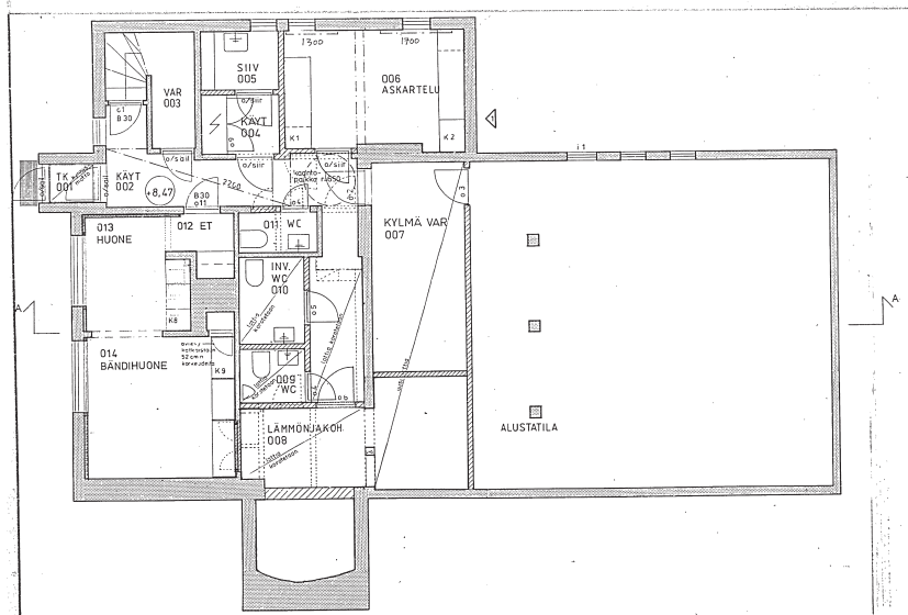
Muutossuunnitelma, kellarikerros. ESA.
