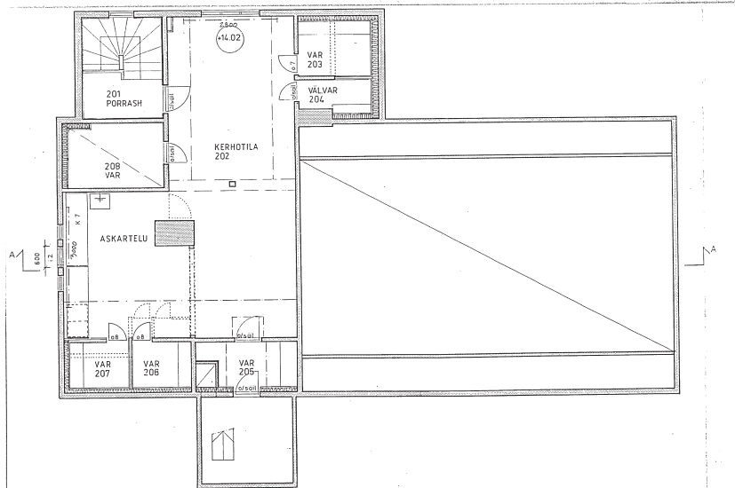
Muutossuunnitelma, 2. kerros. ESA.
