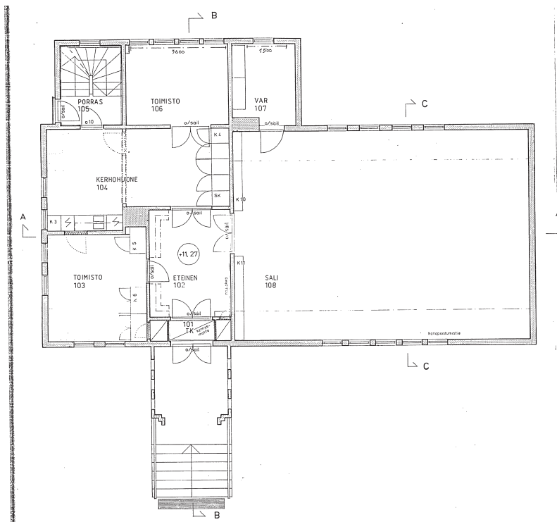
Muutossuunnitelma, 1. kerros. ESA.
