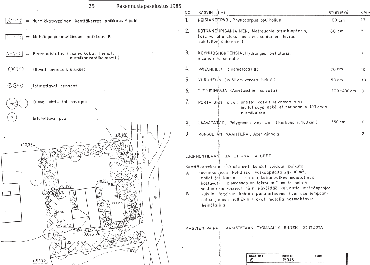
Arkkitehtitoimisto Kaisa ja Jussi Vepsäläisen vihersuunnitelma vuodelta 1985. ESA.
