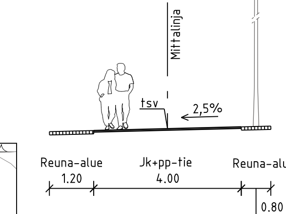
TYYPPIPOIKKILEIKKAUS B-B 1:100
