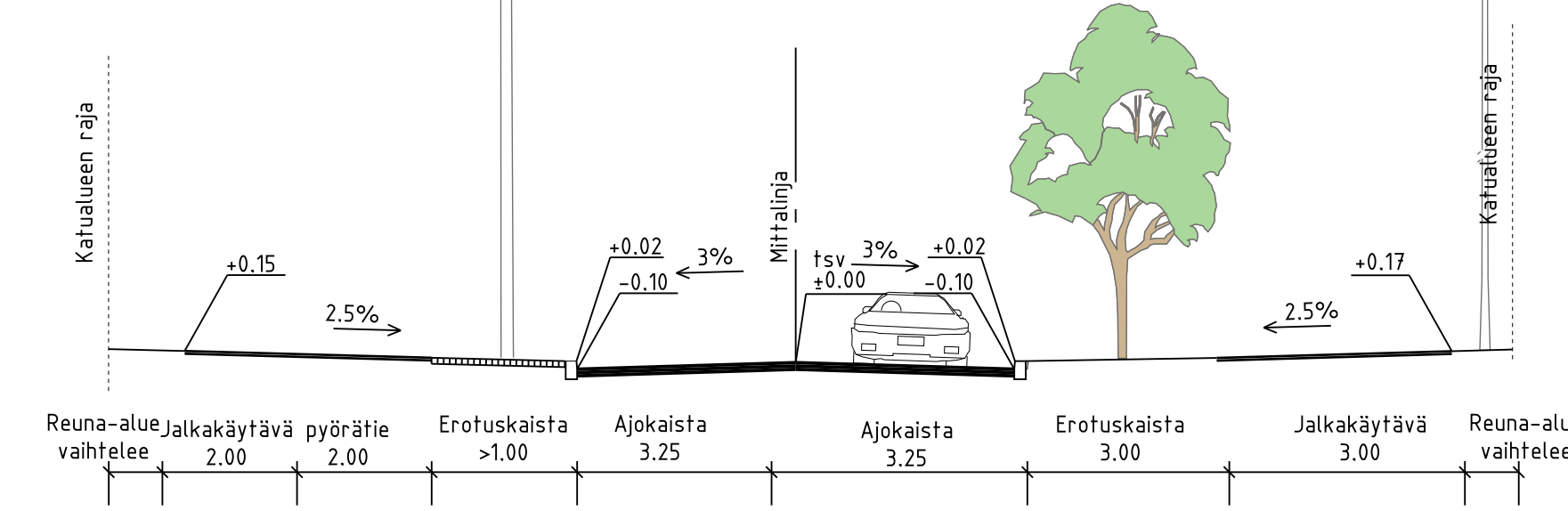
TYYPPIPOIKKILEIKKAUS A-A 1:100
