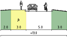
Sävelharju C-C
