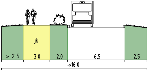
Paciuskentie B-B
