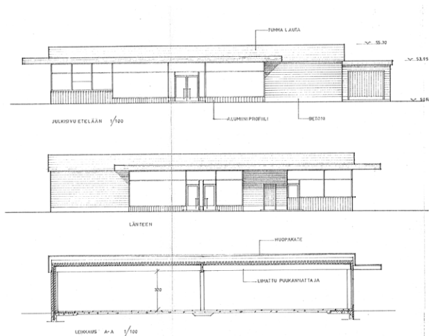
Myymän julkisivupiirustukset on laatinut Kulutusosuuskuntien Keskusliiton arkkitehtiosasto. (Espoon rakennusvalvonta)
