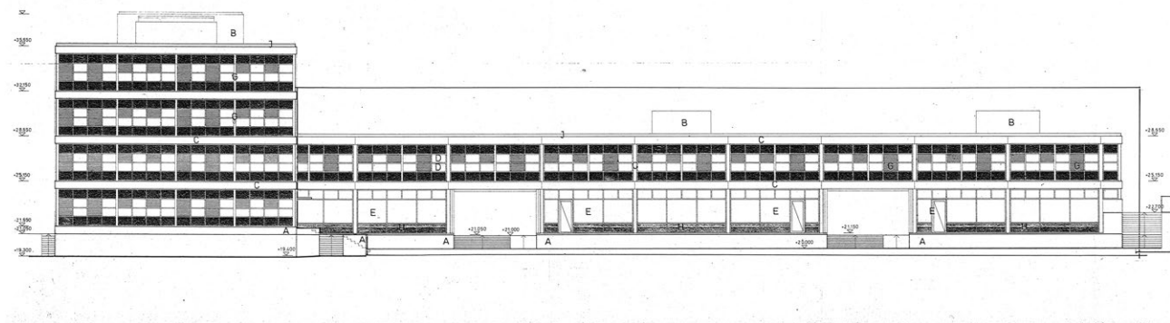
Kuunkierros 4:n julkisivupiirros etelään vuodelta 1974. (Espoon rakennusvalvonta)
