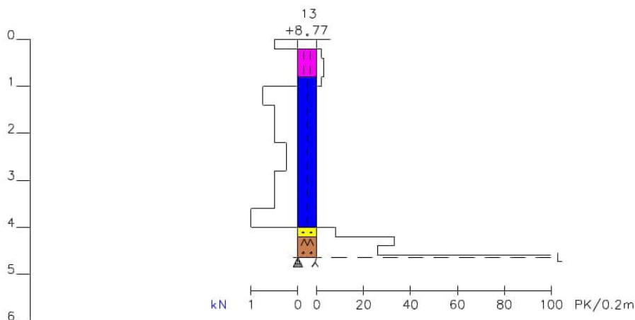
Kuva 2: Ympyröidyn kairauksen diagrammi (huom. ei mittakaavassa)
