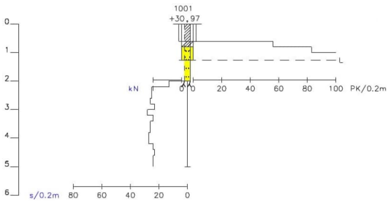
Kuva 3: Ympyröidyn kairauksen diagrammi (huom. ei mittakaavassa)
