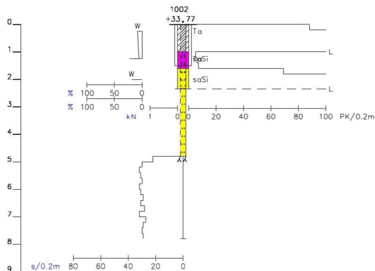
Kuva 5: Ympyröidyn kairauksen diagrammi (huom. ei mittakaavassa)
