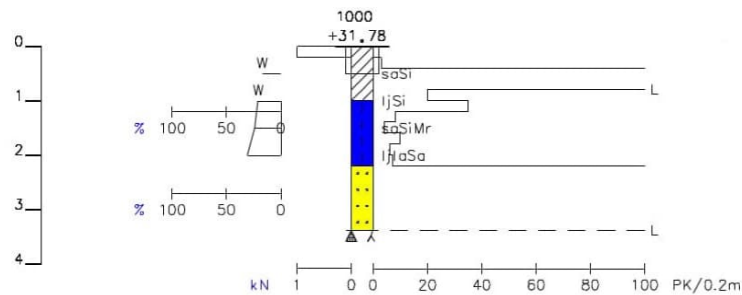
Kuva 4: Ympyröidyn kairauksen diagrammi (huom. ei mittakaavassa)
