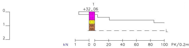
Kuva 2: Ympyröidyn kairauksen diagrammi (huom. ei mittakaavassa)
