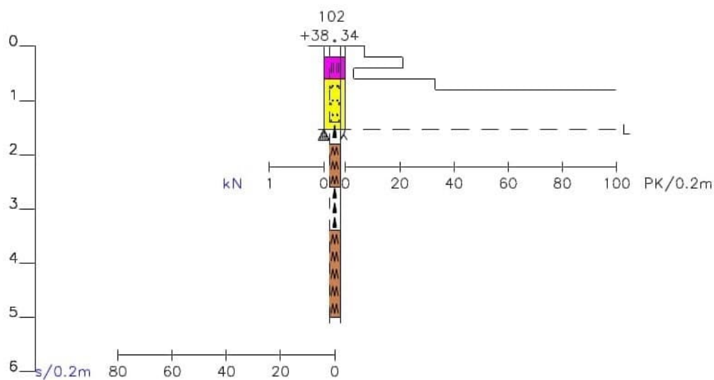
Kuva 2: Ympyröidyn kairauksen diagrammi (huom. ei mittakaavassa)
