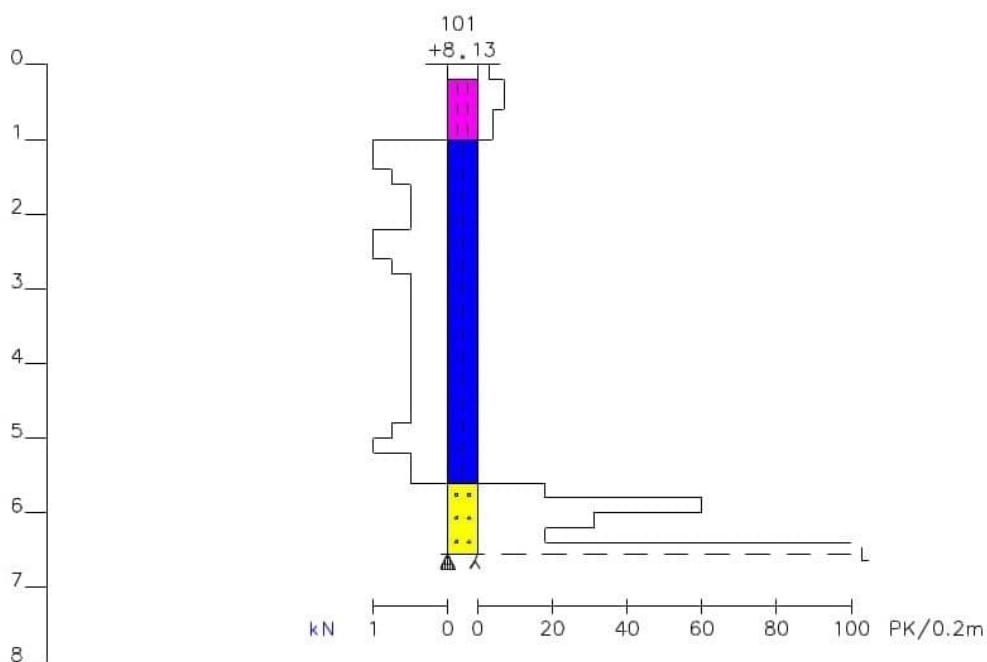
Kuva 2: Ympyröidyn kairauksen diagrammi (huom. ei mittakaavassa)
