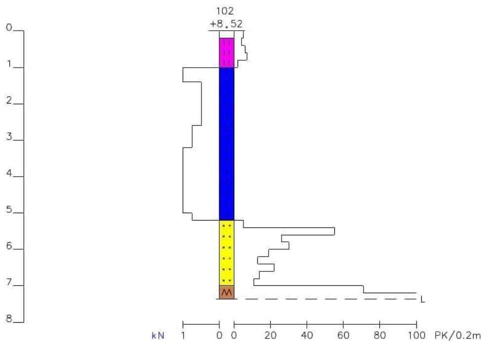
Kuva 2: Ympyröidyn kairauksen diagrammi (huom. ei mittakaavassa)
