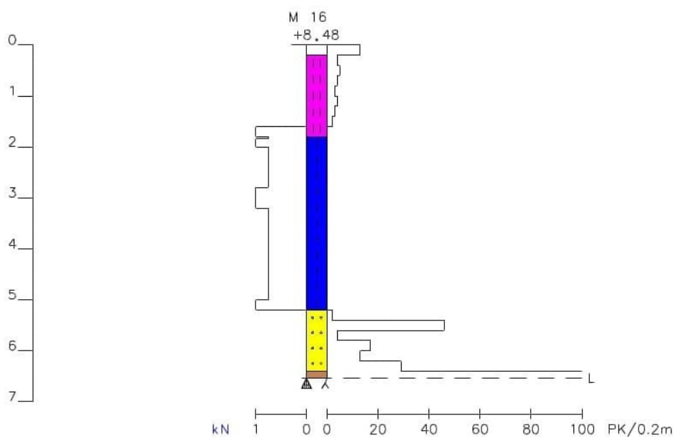
Kuva 2: Ympyröidyn kairauksen diagrammi (huom. ei mittakaavassa)
