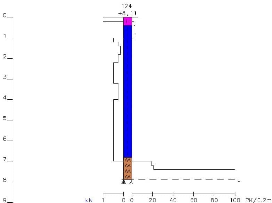
Kuva 2: Ympyröidyn kairauksen diagrammi (huom. ei mittakaavassa)
