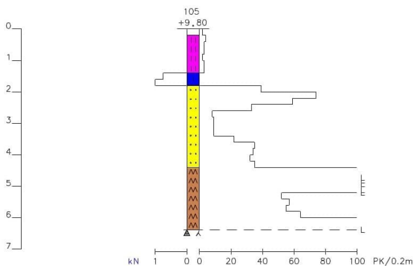
Kuva 2: Ympyröidyn kairauksen diagrammi (huom. ei mittakaavassa)
