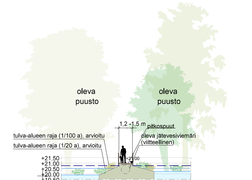
LEIKKAUS CC', 1:200
