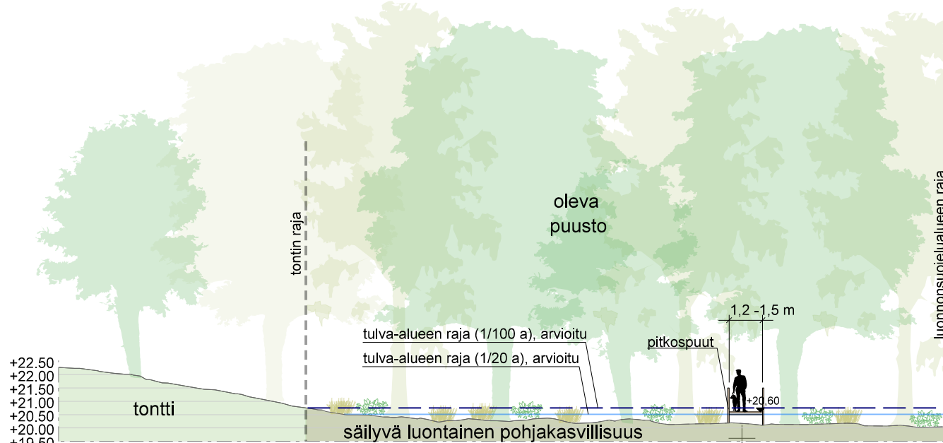
LEIKKAUS BB', 1:200
