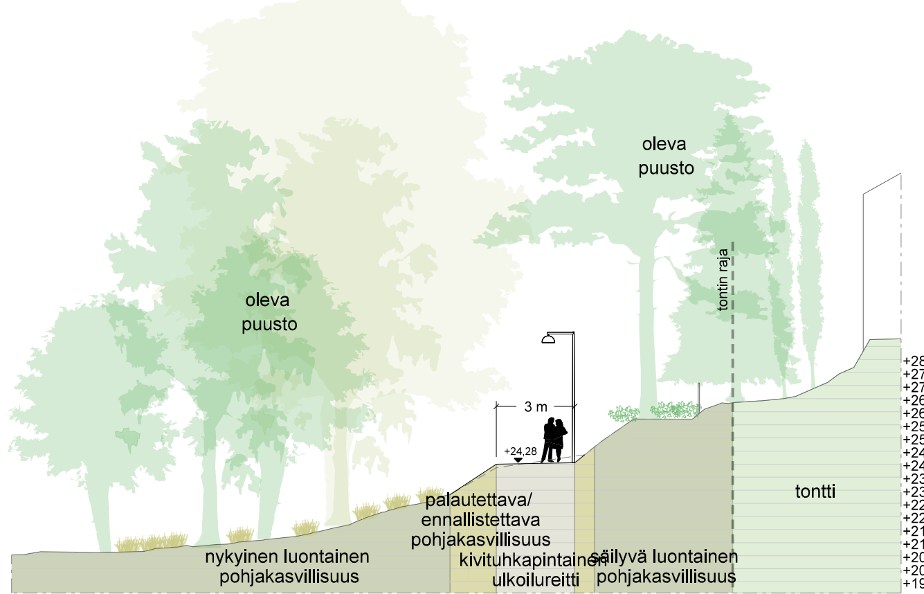
LEIKKAUS AA', 1:200
