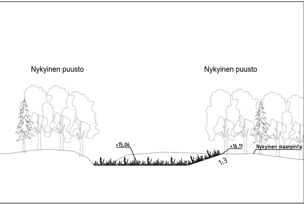
TYYPPIPOIKKILEIKKAUS B-B, 1:200
