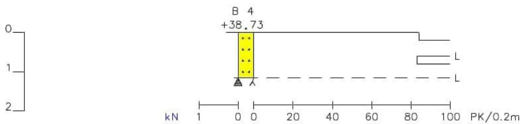
Kuva 2: Ympyröidyn kairauksen diagrammi (huom. ei mittakaavassa)
