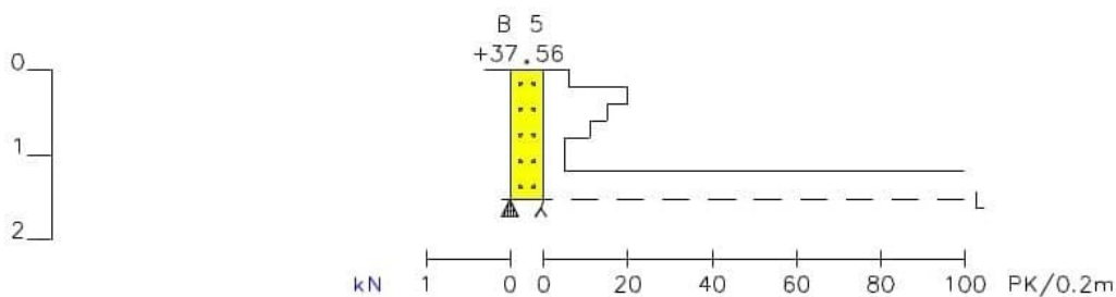
Kuva 2: Ympyröidyn kairauksen diagrammi (huom. ei mittakaavassa)
