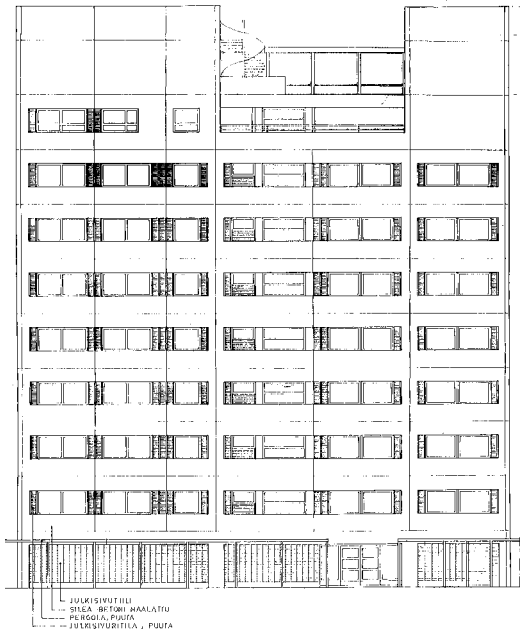
Marintornit rakennuslupakuva, Asuntosäätiö suunnitteluosasto 20.1.1973, 15.4.1973, julkisivu luoteeseen
