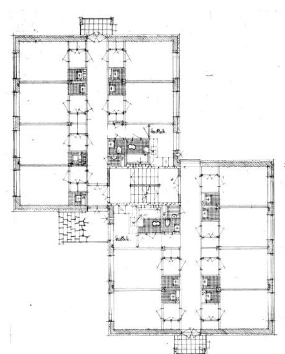
Pohjapiirros. Erich von Ungern -Sternberg 1956. Tilakeskus
