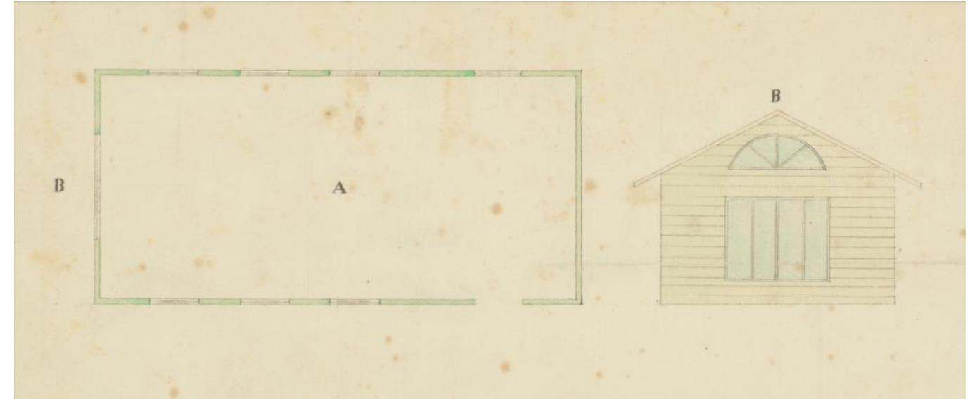
Ajoittamaton kasvihuonepiirustus on mahdollisesti puutarhuri C.J. Helmin laatima. Rakennuksen koko on n. 6 m x 13,2 m (10 x 22 kyyn.) Museovirasto
