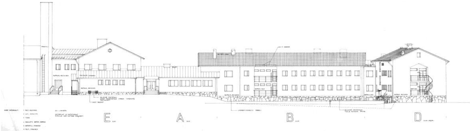
A-E julkisivut kaakkoon ja luoteeseen 1990-luvun vaihteessa. Tilakeskus arkisto
