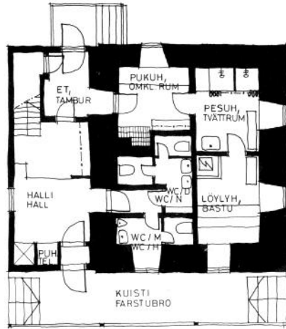
Kuva 62. Pesutuvan 1. kerros 1:100.
