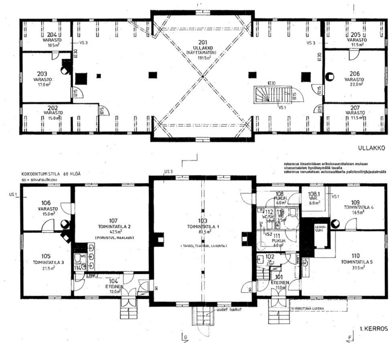
1. ja 2. kerros. Korjaustyön pääpiirustus Arkkitehtitoimisto Nurmela Raimoranta Tasa 2000. ERVV
