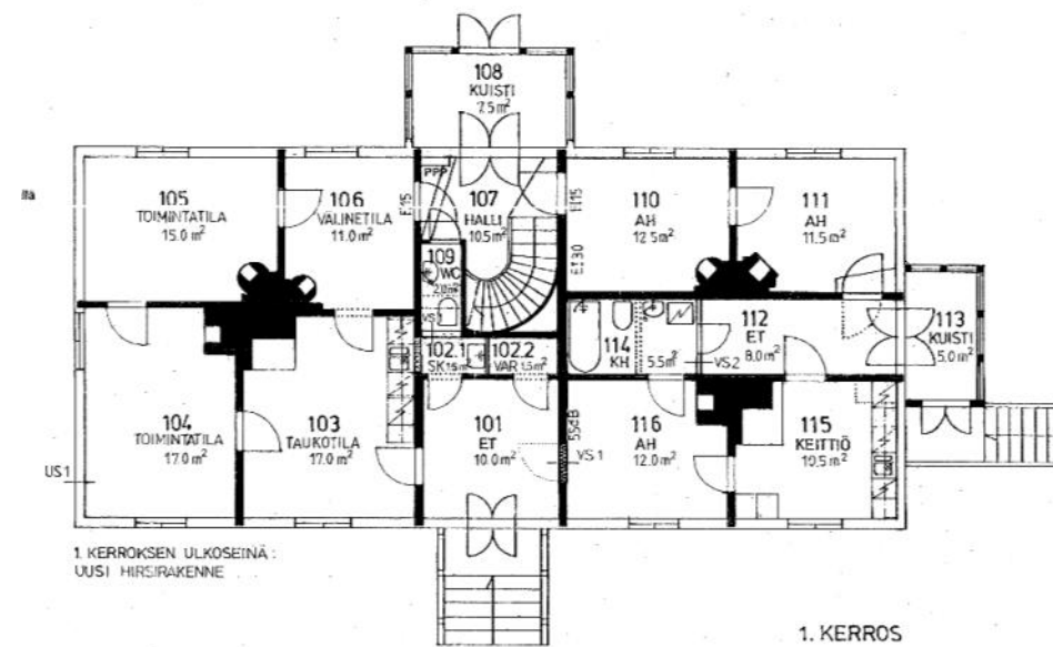
1. ja 2. kerros. Korjaustyön pääpiirustus Arkkitehtitoimisto Nurmela Raimoranta Tasa 2000. ERVV
