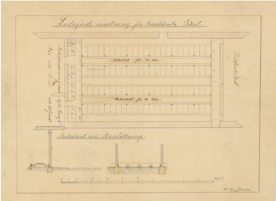
Osapiirros 1885. Alb. Voss-Schrader. Museovirasto
