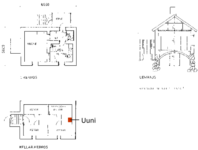
Pohjat, leikkaukset ja julkisivut. Korjaustyön pääpiirustus 1985. Espoon kaupungin tekninen virasto
