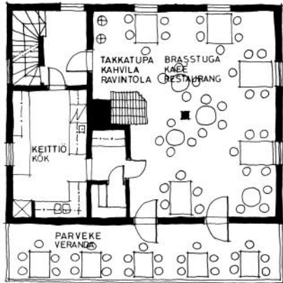
Kuva 61. Pesutuvan 2. kerros 1:100.
