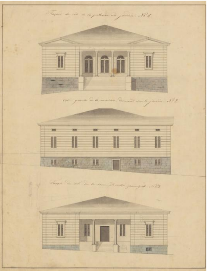
Päärakennus julkisivut kaakkoon, lounaaseen ja luoteeseen. Pohjapiirros johon on merkitty huoneiden käyttö. Museovirasto
