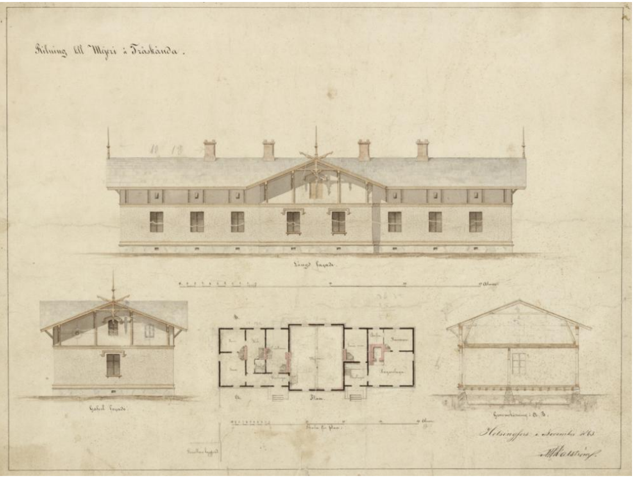
Piirustus marraskuussa 1863, Ritning till Mejeri i Träskända. A.H. Dalström. Museovirasto
