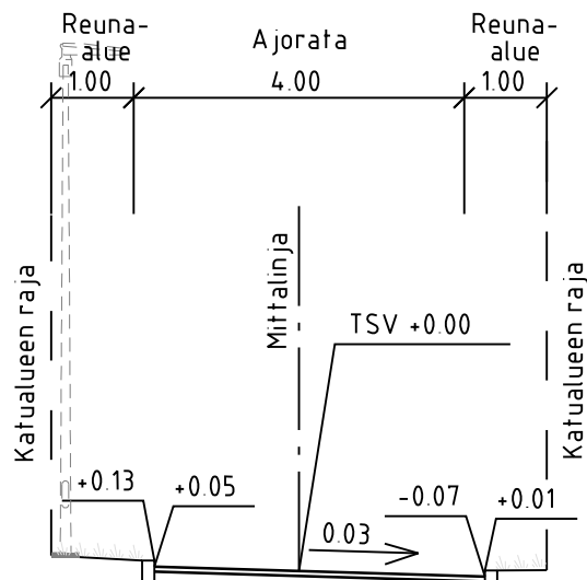
TYYPPIPOIKKILEIKKAUS B-B 1:100
