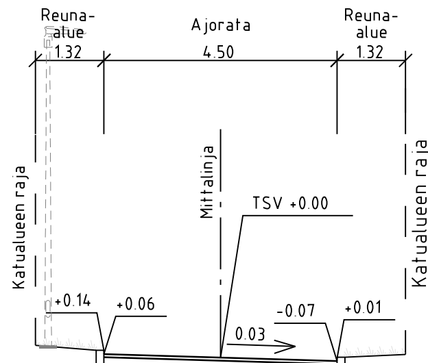
TYYPPIPOIKKILEIKKAUS C-C 1:100
