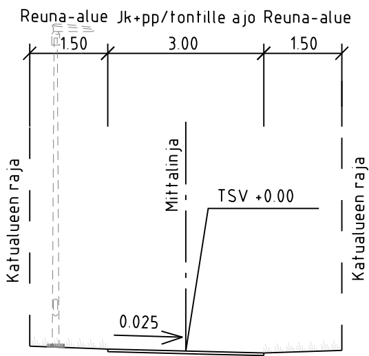
TYYPPIPOIKKILEIKKAUS A-A 1:100
