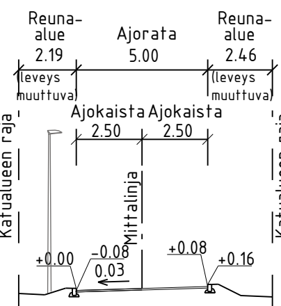
TYYPPIPOIKKILEIKKAUS A-A 1:200
