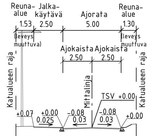
TYYPPIPOIKKILEIKKAUS B-B 1:200
