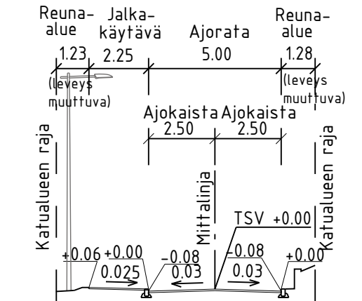
TYYPPIPOIKKILEIKKAUS A-A 1:200
