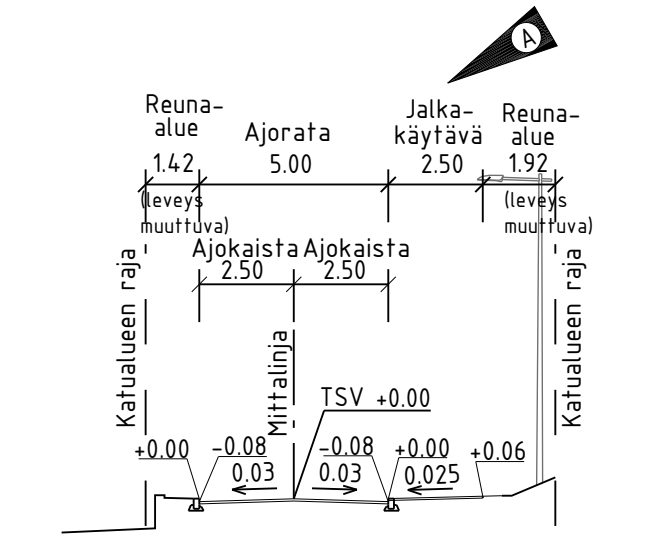
TYYPPIPOIKKILEIKKAUS A-A 1:200
