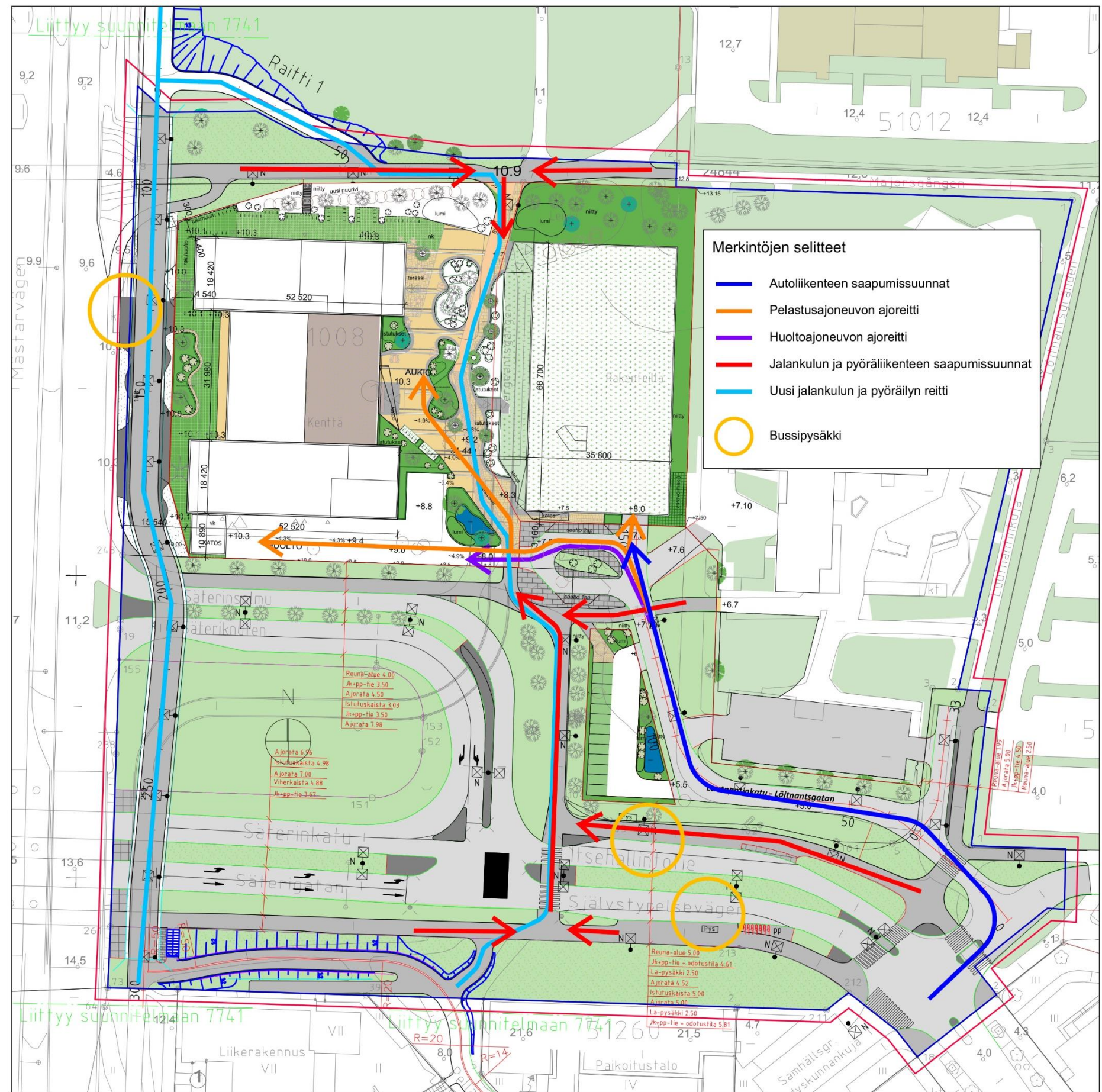
LIIKENNESUUNNITELMAKAAVIO
