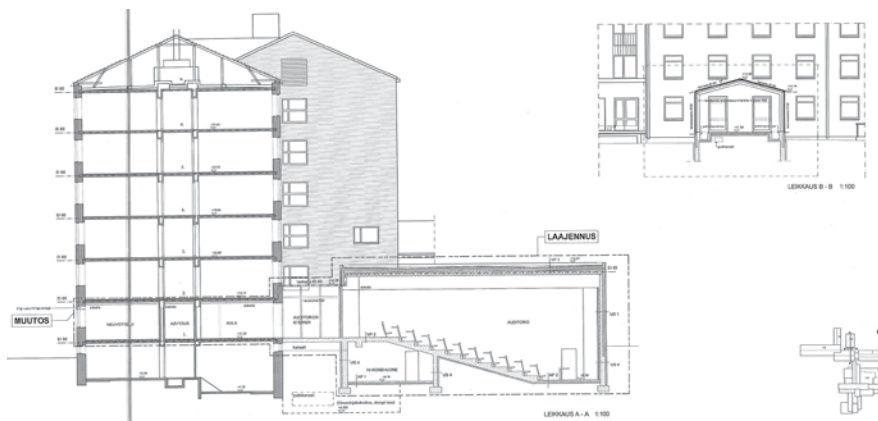
Auditoriosiiven leikkauspiirustus pohjoiseen sekä lasi-teräsrakenteisen yhdysosan poikkileikkaus. 30.9.2003. Arkkitehtitoimisto Jukka Turtiainen. ERava.
