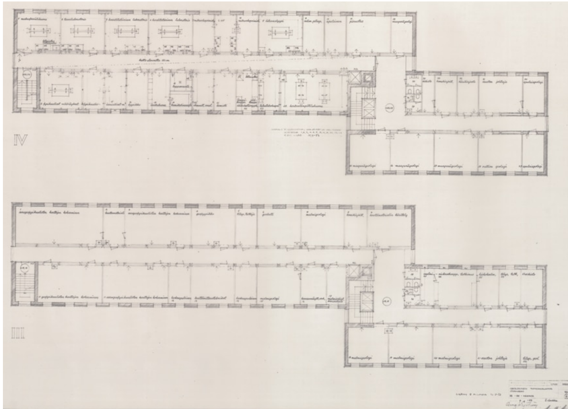
Neljännen ja viidennen kerroksen pohjapiirustus. Rakennushallitus. E. Larkka 9.4.1953. KA.
