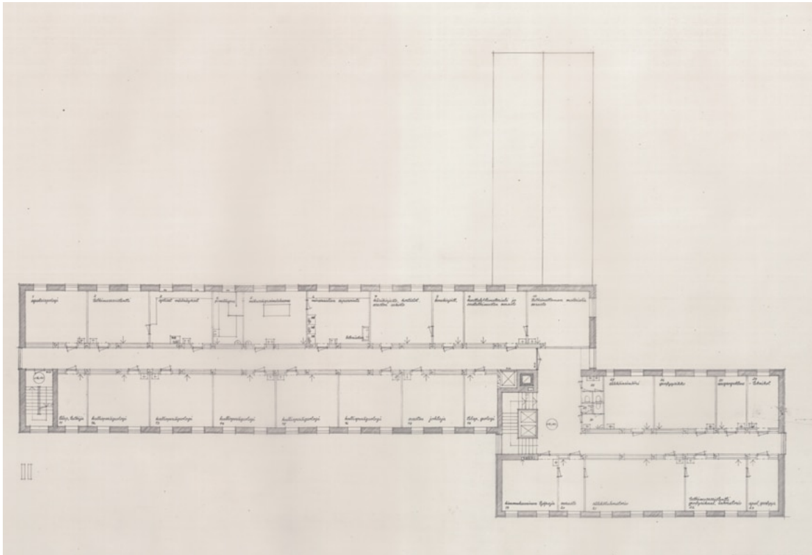
Toisen kerroksen pohjapiirustus. Rakennushallitus. E. Larkka 9.4.1953. KA.
