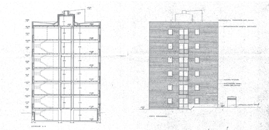
Laajennuksen leikkauspiirustus ja pohjoisjulkisivupiirustus. 9.5.1968. Tuula Vainio. ERava.
