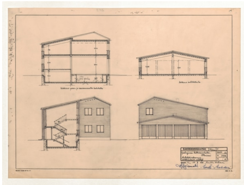
Autotallirakennuksen eteläjulkisivu- ja leikkauspiirustus. Rakennushallitus. Annikki Virtanen. 2.11.1955. KA.
