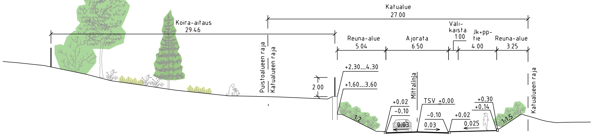
TYYPPIPOIKKILEIKKAUS A-A 1:200
