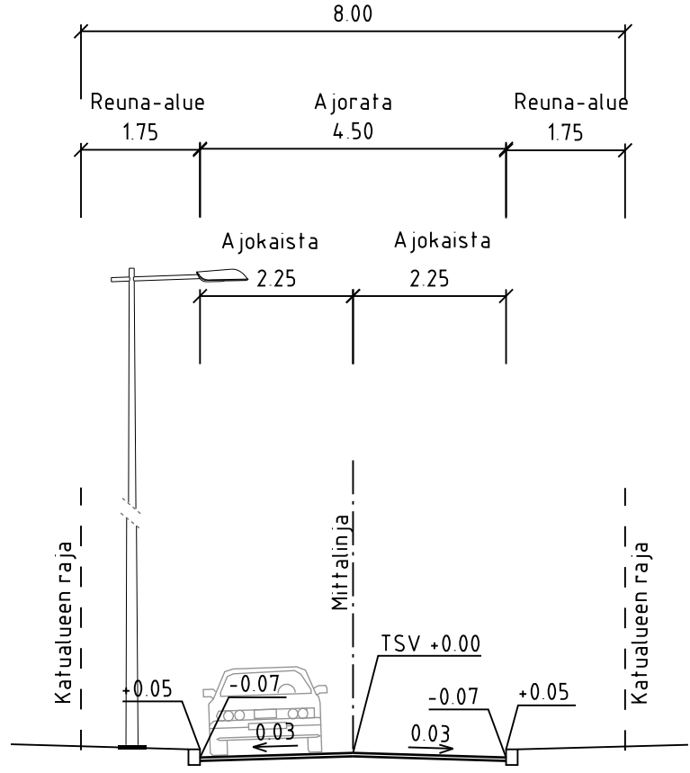
VÄLIKALLIONKUJA TYYPPIPOIKKILEIKKAUS C-C 1:100
