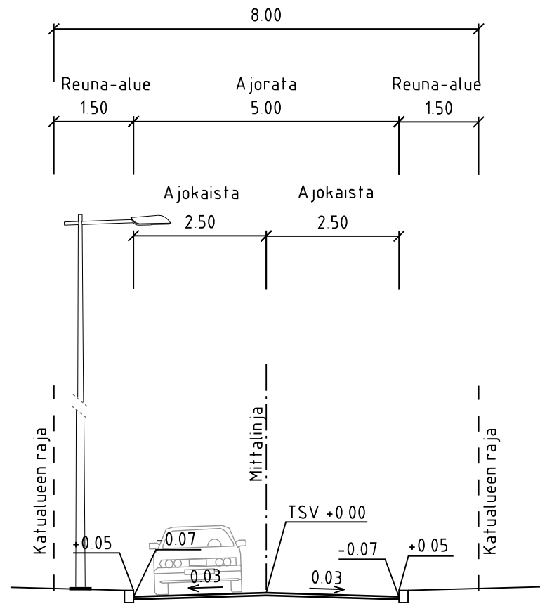
VÄLIKALLIO välillä Gobbackantie-Välikallionkuja TYYPPIPOIKKILEIKKAUS A-A 1:100
