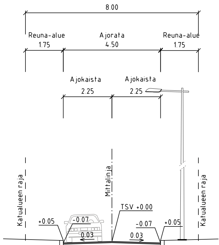
VÄLIKALLIO välillä Välikallionkuja-pl 148 TYYPPIPOIKKILEIKKAUS B-B 1:100
