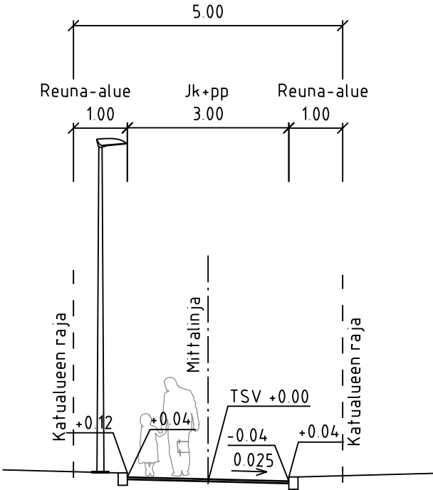
VÄLIKALLIONKUJA Jk+pp-tie TYYPPIPOIKKILEIKKAUS D-D 1:100
