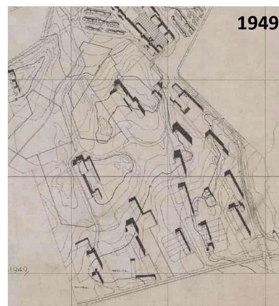
Pitkälti kilpailuehdotukseen perustuvassa vuoden 1949 maankäyttösuunnitelmassa on massoitellutaan puikkomaiset rakennukset sijoitettu viuhkamaisesti ja maaston muotoja mukaillen.
