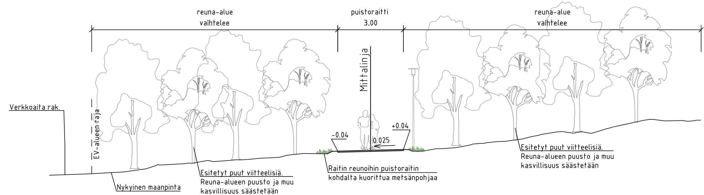
TYYPPIPOIKKILEIKKAUS A-A 1:100
