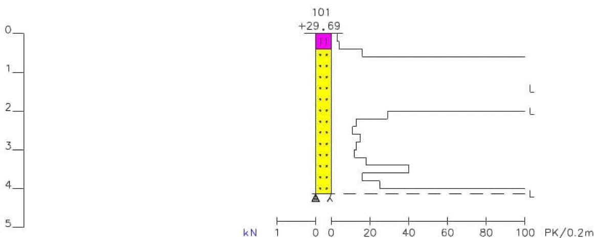
Kuva 2: Ympyröidyn kairauksen diagrammi (huom. ei mittakaavassa)
