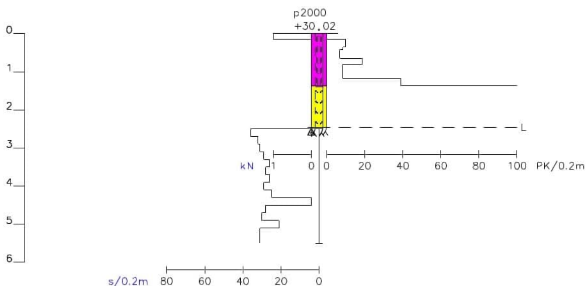
Kuva 2: Ympyröidyn kairauksen diagrammi (huom. ei mittakaavassa)
