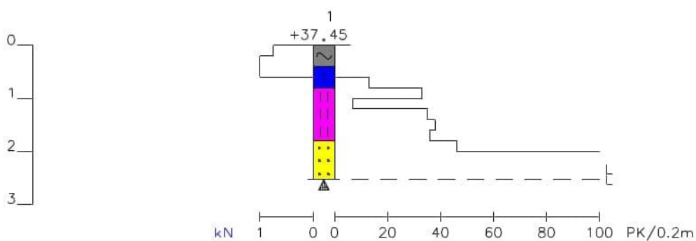
Kuva 2: Ympyröidyn kairauksen diagrammi (huom. ei mittakaavassa)
