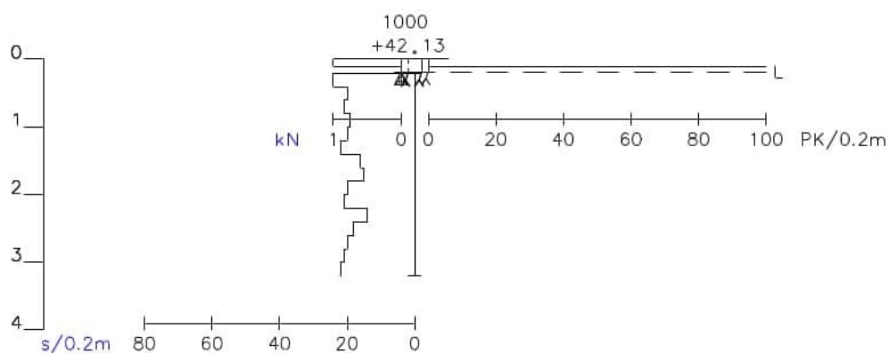
Kuva 2: Ympyröidyn kairauksen diagrammi (huom. ei mittakaavassa)
