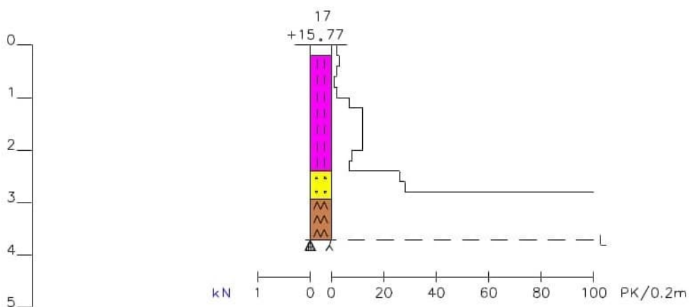
Kuva 2: Ympyröidyn kairauksen diagrammi (huom. ei mittakaavassa)
