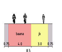
LAAJALAHDENBAANA (vain siltataso esitetty), LEIKKAUS G - G
