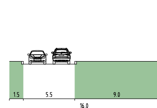
LUUTNANTINKATU, LEIKKAUS E - E
