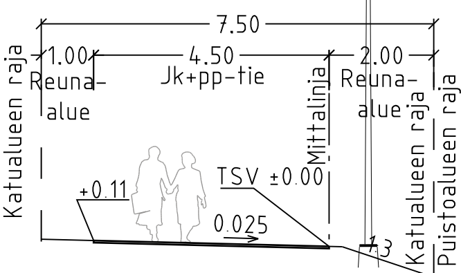
TYYPPIPOIKKILEIKKAUS A-A 1:100
