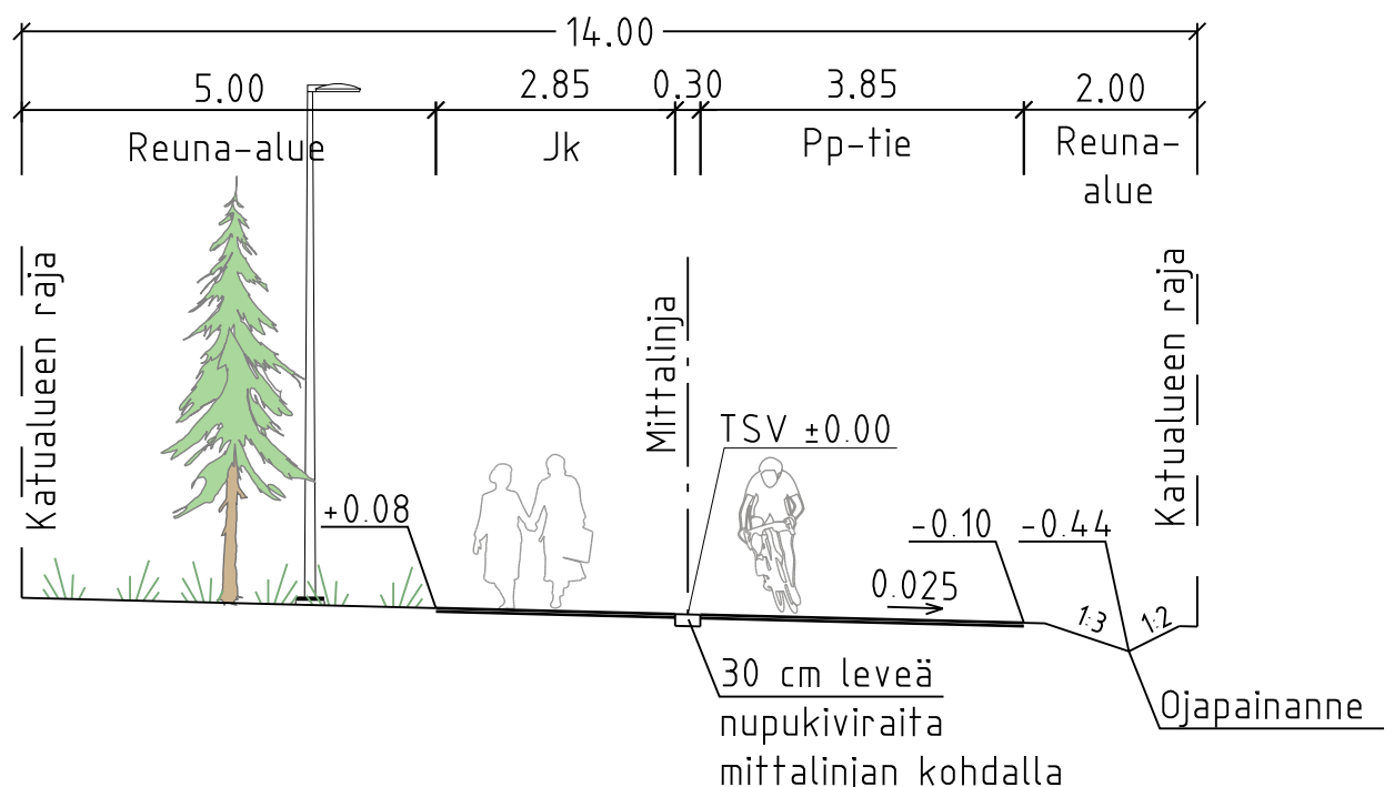
TYYPPIPOIKKILEIKKAUS A-A 1:100
