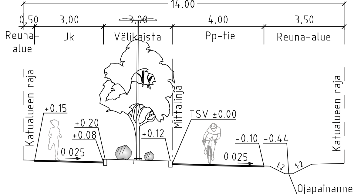
TYYPPIPOIKKILEIKKAUS B-B 1:100
