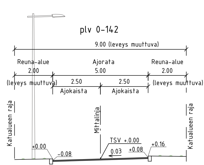
TYYPPIPOIKKILEIKKAUS A-A 1:100
