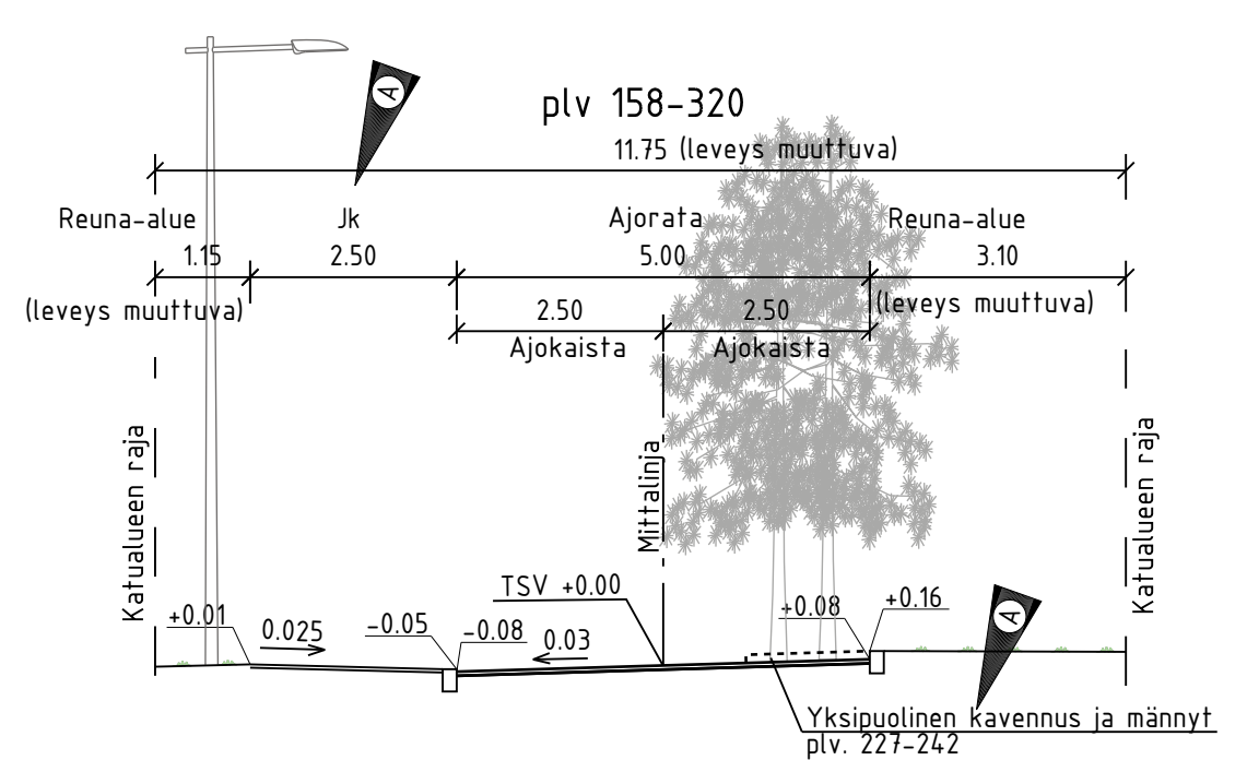
TYYPPIPOIKKILEIKKAUS B-B 1:100
