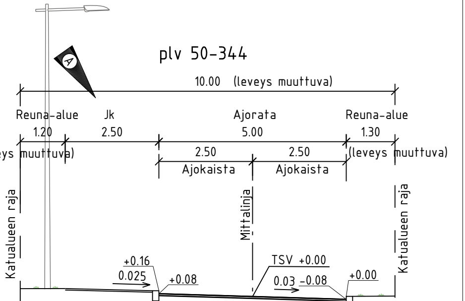
TYYPPIPOIKKILEIKKAUS B-B 1:100
