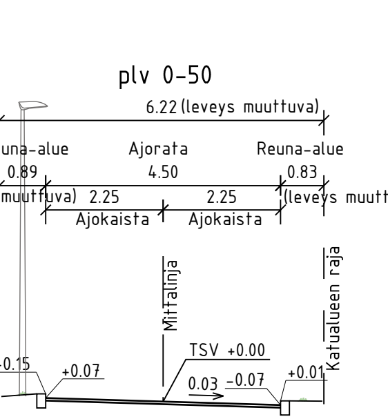
TYYPPIPOIKKILEIKKAUS A-A 1:100
