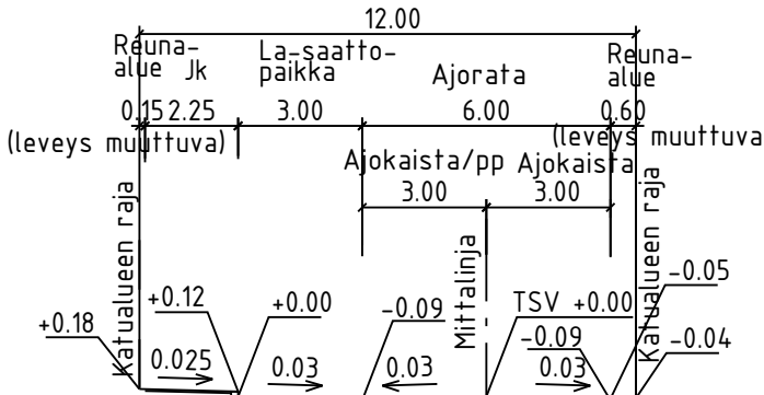
TYYPPIPOIKKILEIKKAUS A-A 1:200
