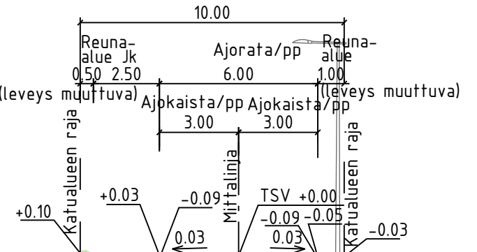
TYYPPIPOIKKILEIKKAUS B-B 1:200
