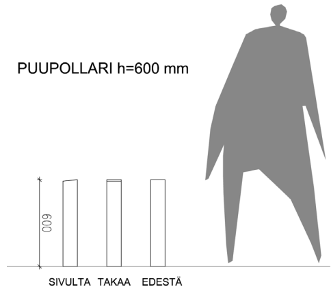
Puupollari, 100 x 100 mm painekyllästetty sahatavara, korkeus 600 mm, kuultokäsittely kahteen kertaan tumman ruskeaksi (TVT 5728). (Aita ja pollari Tapiolaa varten, tyyppipiirustus. Hyväksytty luonnos TDM:ia varten 6.11.2015)
