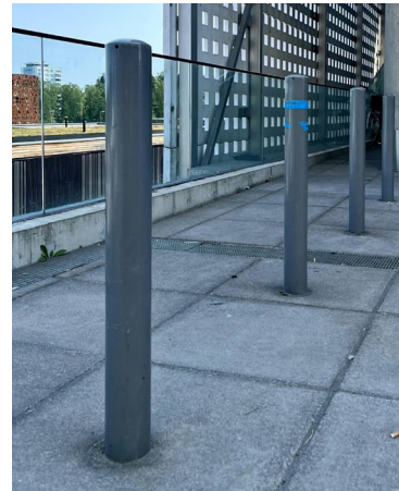
Teräspollareita sijoitettuna Länsituulen itäpäähän. Korkeus 750mm, läpimitta 160mm, RAL 9007.
