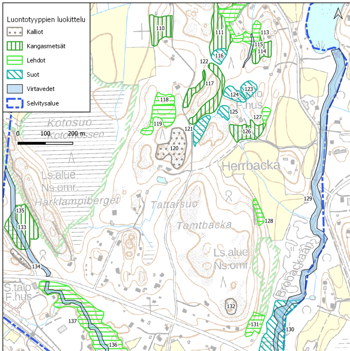
Kuva 32. Stormbackan uhanalaiset luontotyyppit 110–127 ja Herrbackan luontotyyppit 128–131 sekä Nupurinjärveä lähinnä olevat luontotyyppit 133–137.
