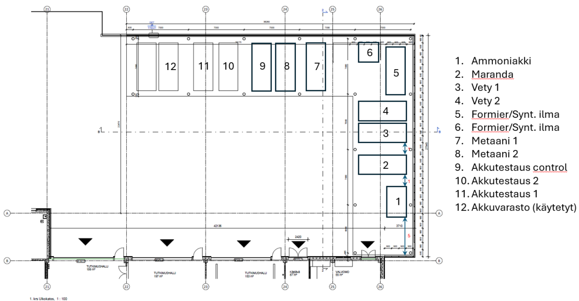
Kuva 11A.2. Konttien sijoittelu konttivarastossa (katos).
